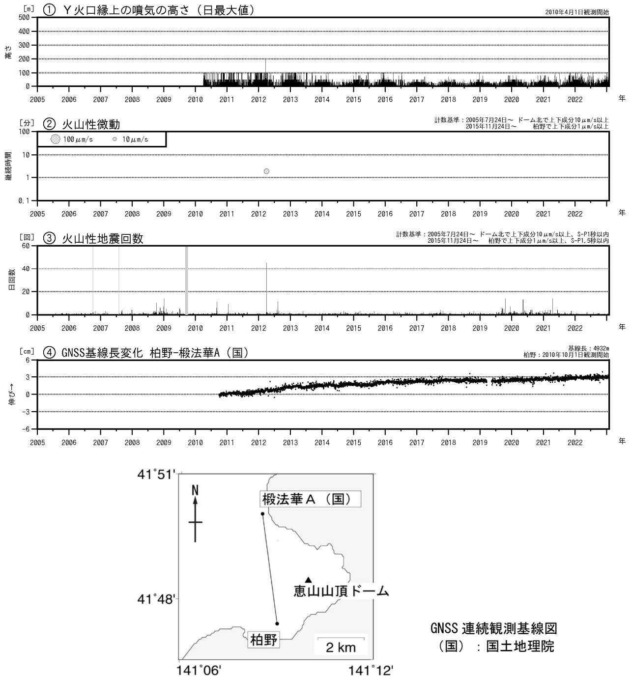
図2 恵山 火山活動経過図（2005年7月～2023年1月） ③の灰色部分は機器障害による欠測期間を示します。 ④のグラフは上図の基線に対応しています。 ④のグラフの空白部分は欠測を示します。
