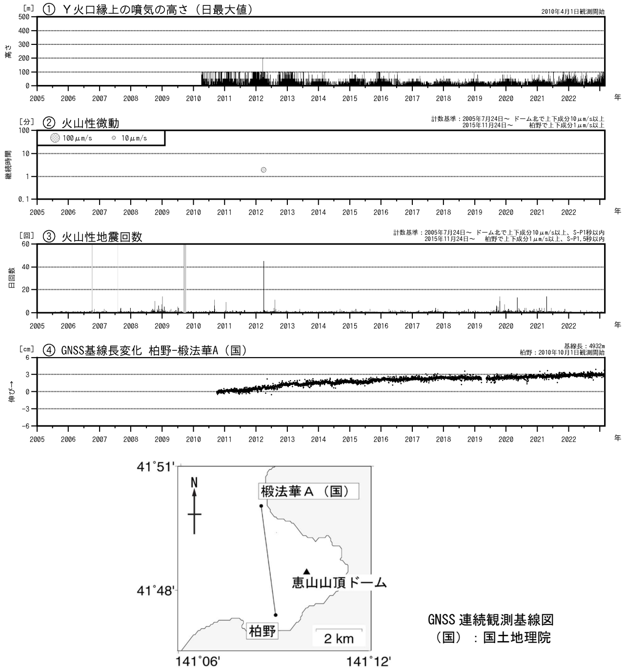
図2 恵山 火山活動経過図（2005年7月～2023年2月） ③の灰色部分は機器障害による欠測期間を示します。 ④のグラフは上図の基線に対応しています。 ④のグラフの空白部分は欠測を示します。
