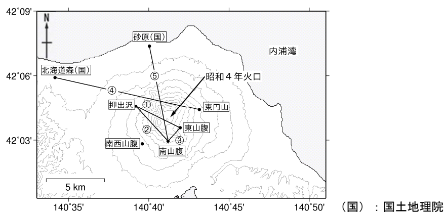
図5 北海道駒ヶ岳 GNSS連続観測による基線長変化（2001年4月～2023年3月）及び観測点配置図 グラフ①～⑤は観測点配置図の基線①～⑤に対応しています。 グラフの空白部分は欠測を示します。
