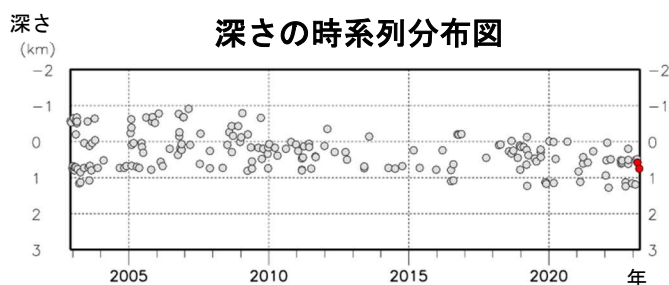
図4 北海道駒ヶ岳 火山性地震の震源分布（2002年12月～2023年3月）
