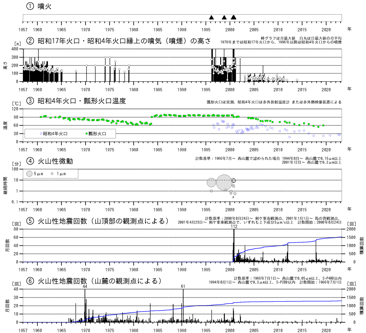
図1 北海道駒ヶ岳 火山活動経過図（1957年1月～2023年3月）
