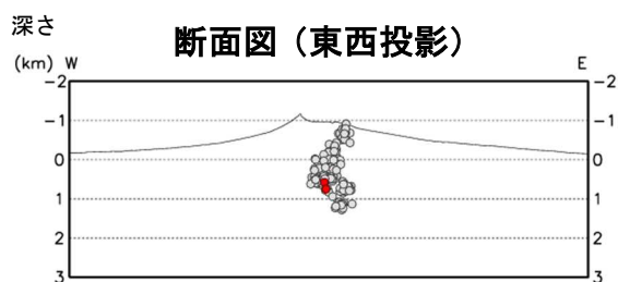
図4 北海道駒ヶ岳 火山性地震の震源分布（2002年12月～2023年3月）
