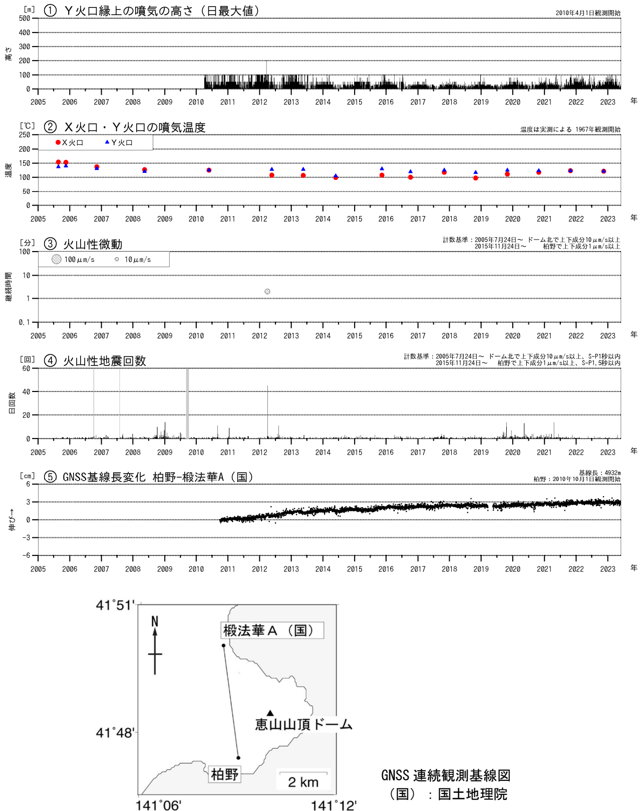
図2 恵山 火山活動経過図（2005年7月～2023年5月） ④の灰色部分は機器障害による欠測期間を示します。 ⑤のグラフは上図の基線に対応しています。 ⑤のグラフの空白部分は欠測を示します。
