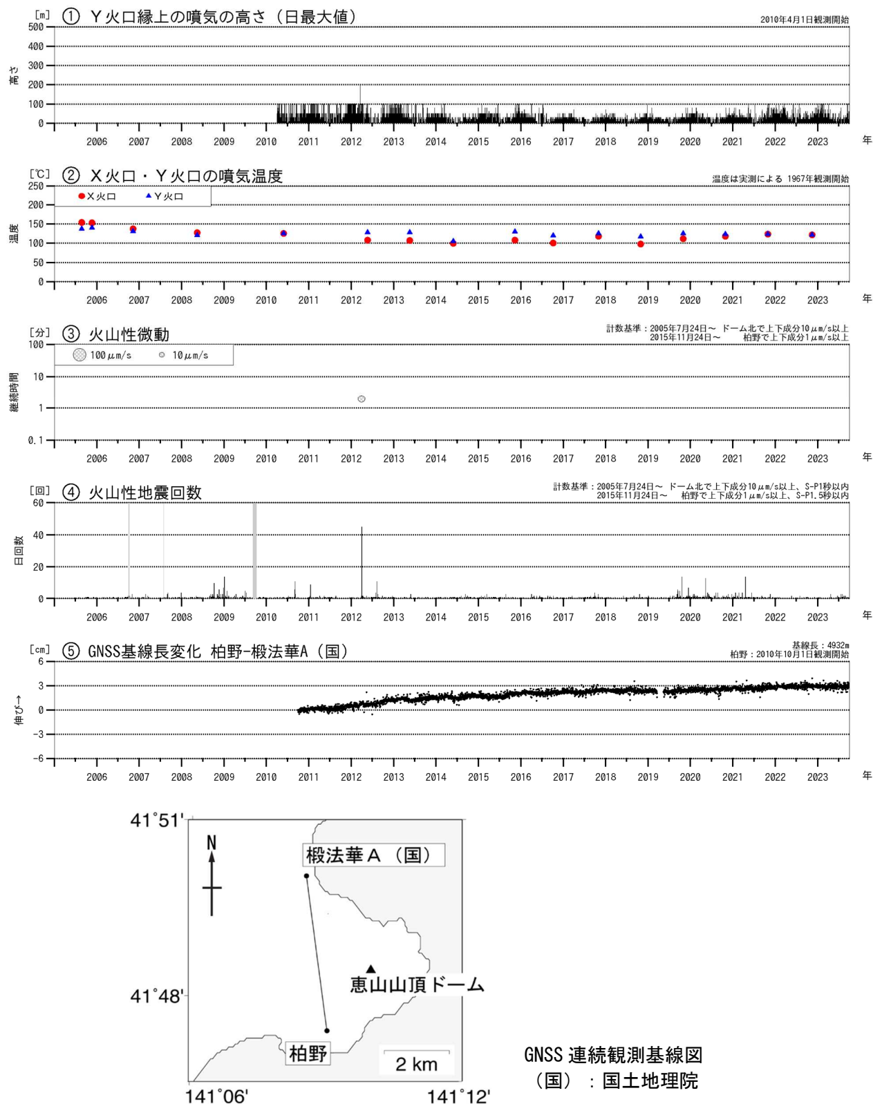
図4 恵山 火山活動経過図（2005年7月～2023年9月） ④の灰色部分は機器障害による欠測期間を示します。 ⑤のグラフは上図の基線に対応しています。 ⑤のグラフの空白部分は欠測を示します。
