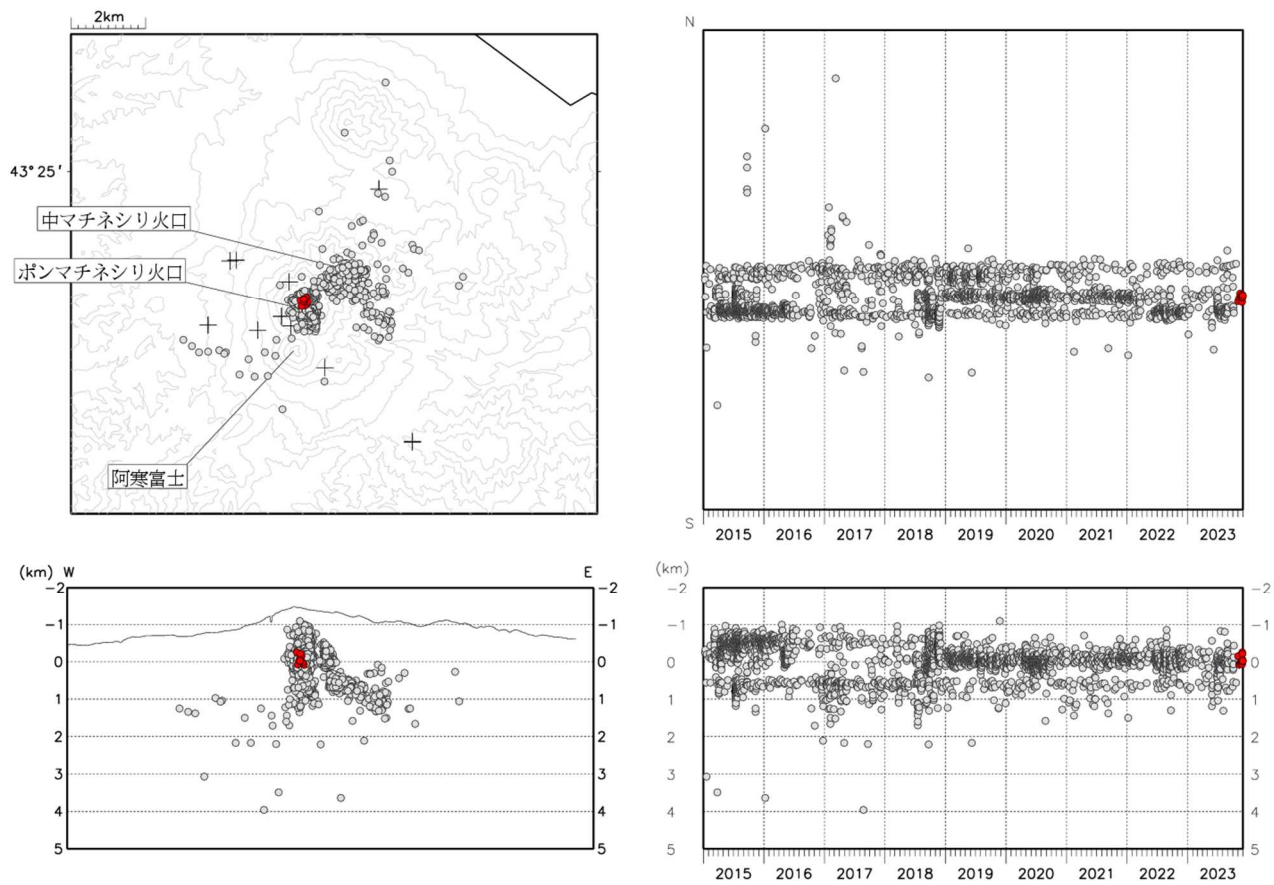
図5 雌阿寒岳 火山性地震の震源分布（2015年1月～2023年11月）
