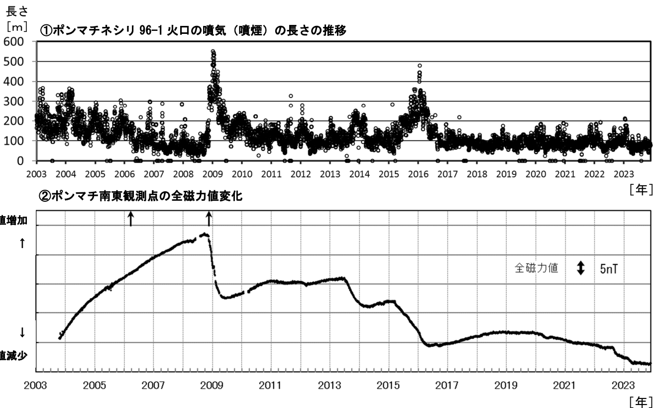
図4 雌阿寒岳 ポンマチネシリ96-1火口の噴気（噴煙）の長さ、全磁力値の経過及び全磁力観測点配置図（2003年～2023年11月）
