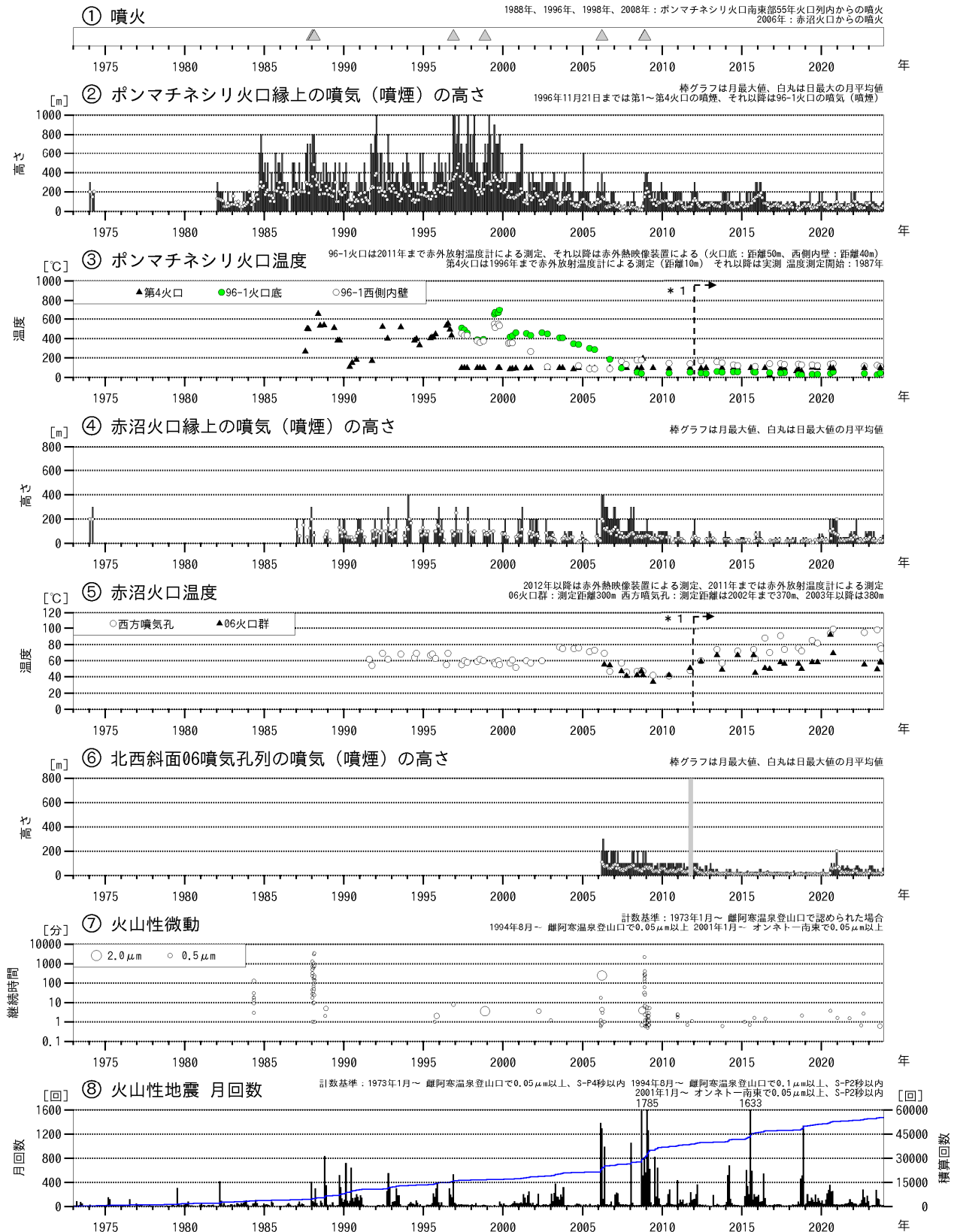
図1 雌阿寒岳 火山活動経過図（1973年1月～2023年11月）
