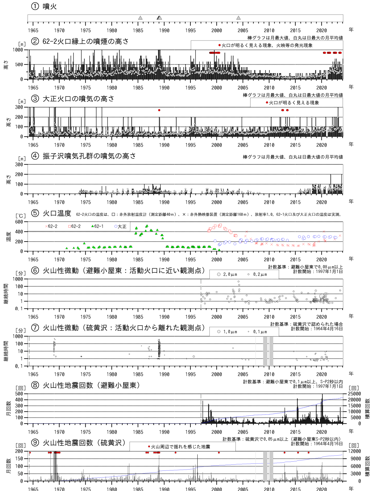
図1 十勝岳 火山活動経過図（1964年1月～2024年1月）
