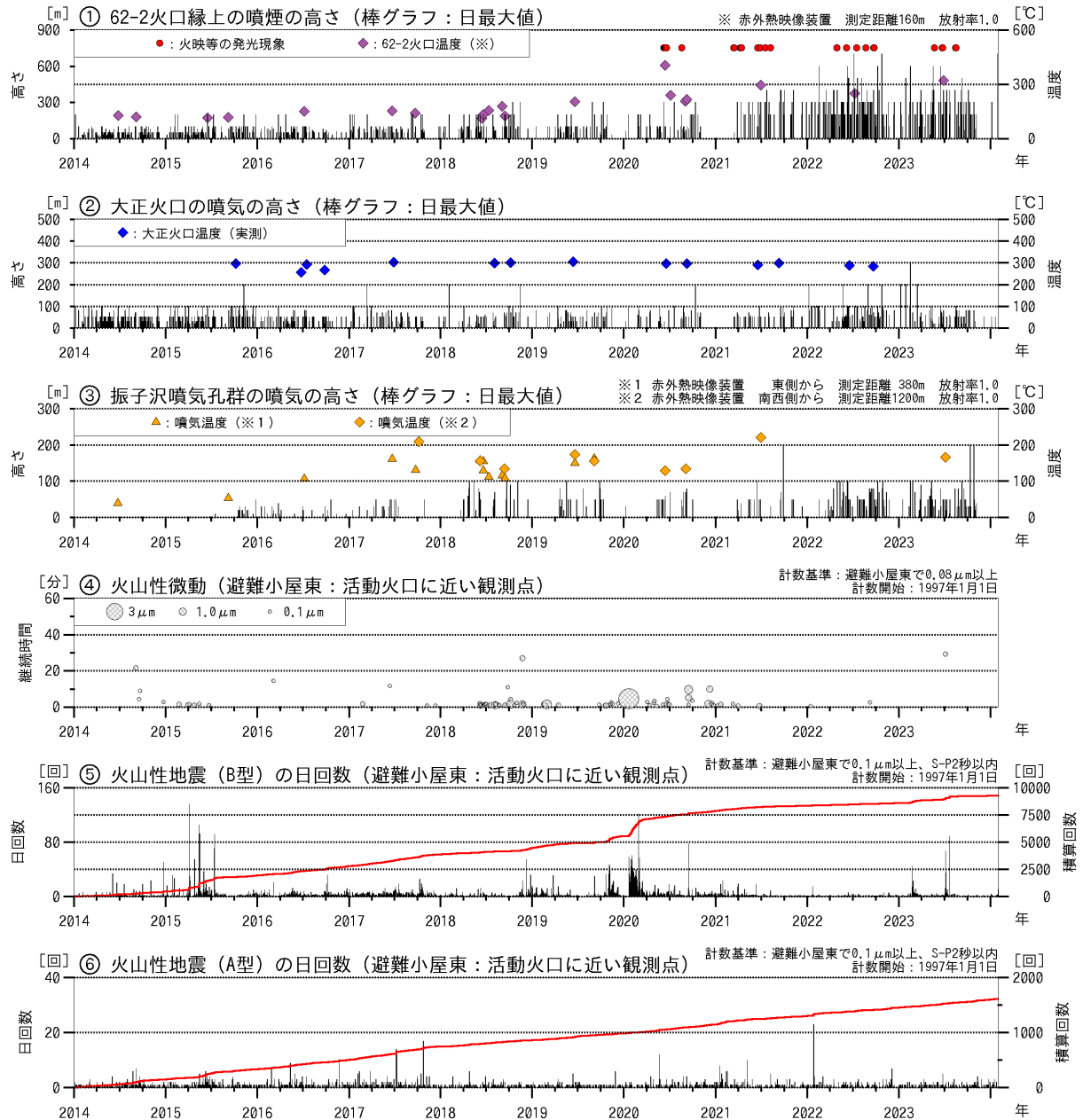
図2 十勝岳 火山活動経過図（2014年1月～2024年1月）
