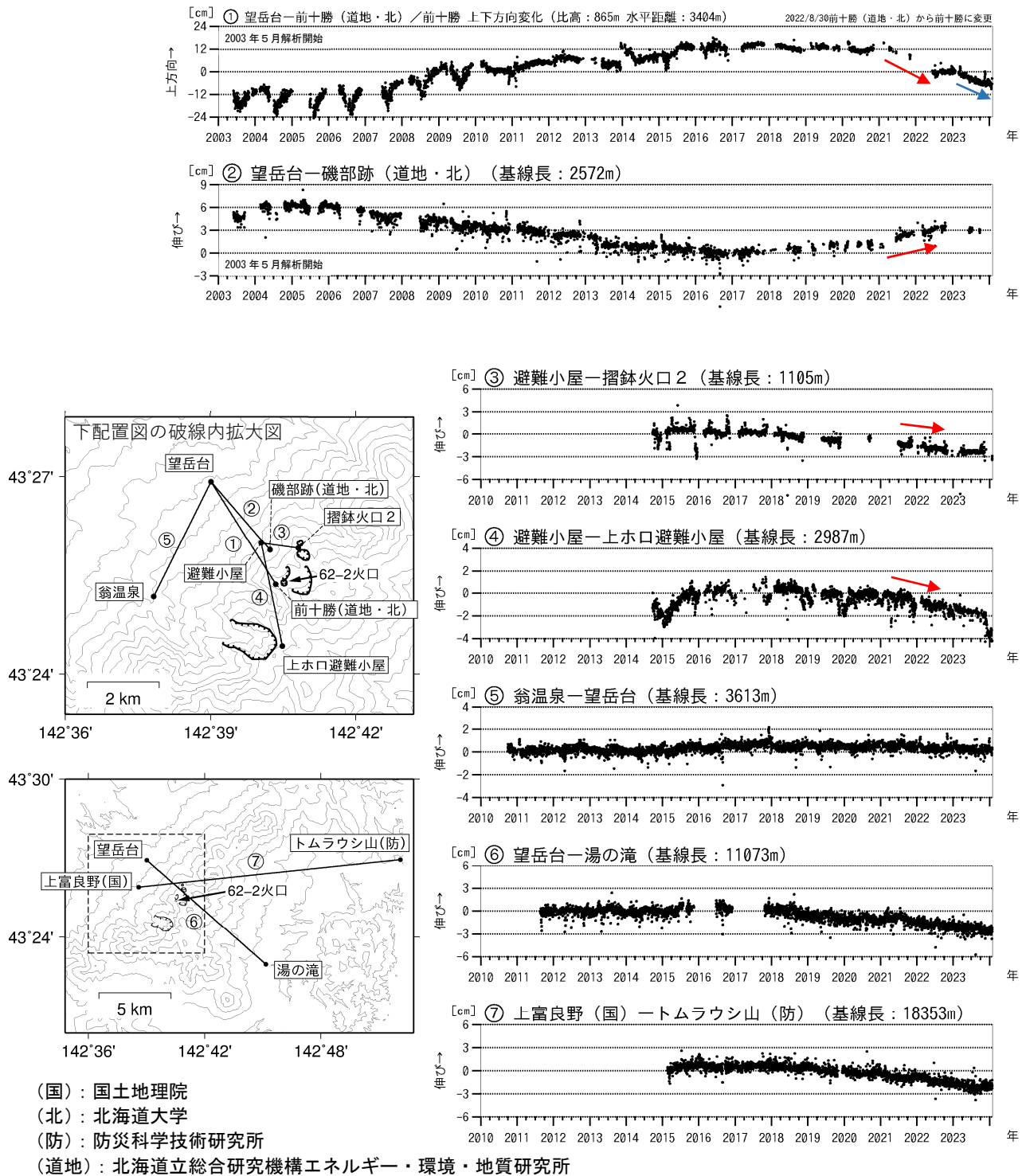
図5 十勝岳 GNSS連続観測による上下方向変化及び基線長変化（2003年5月～2024年1月）及び観測点配置図
