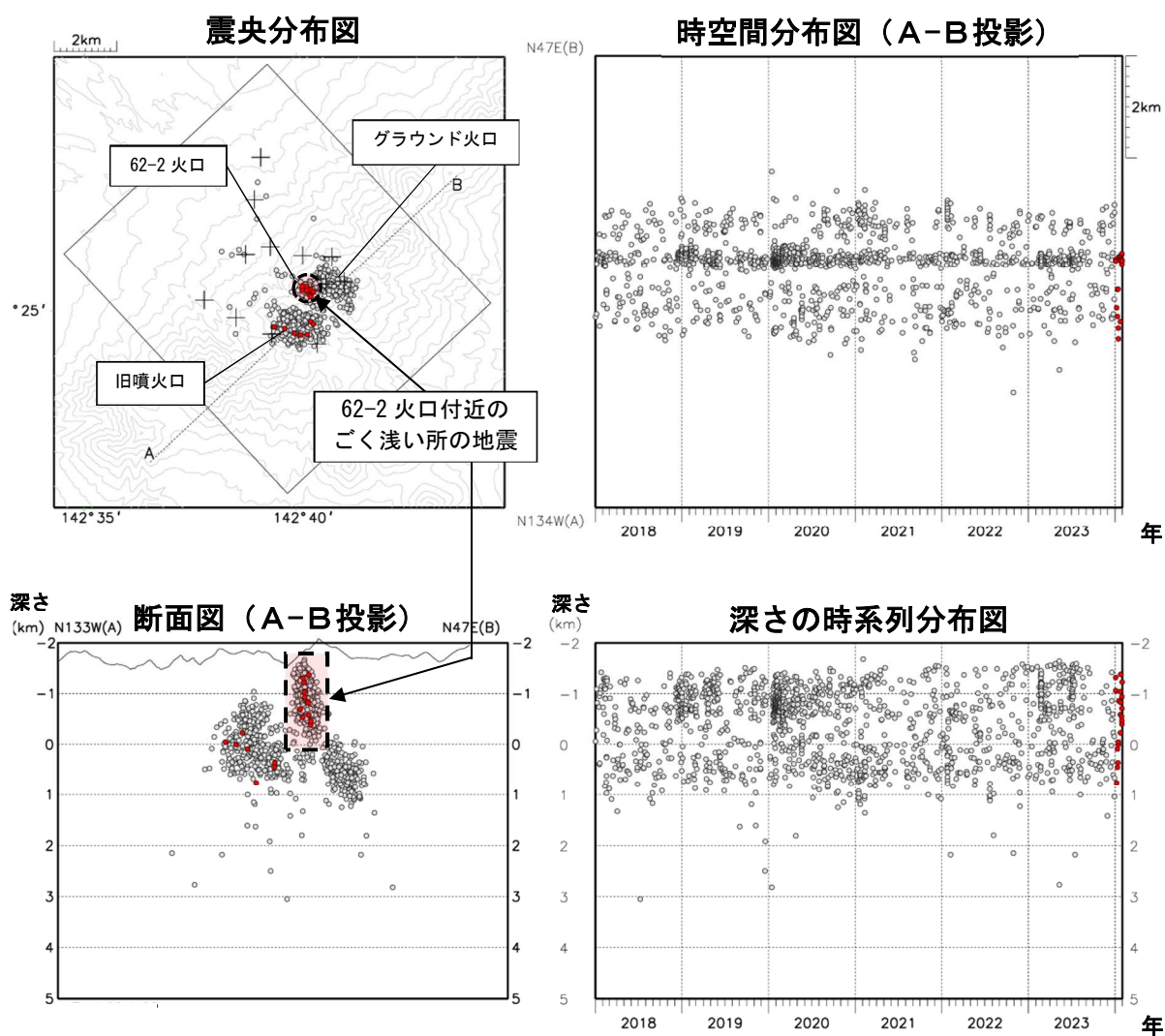
図4 十勝岳 火山性地震の震源分布（2018年1月～2024年1月）
