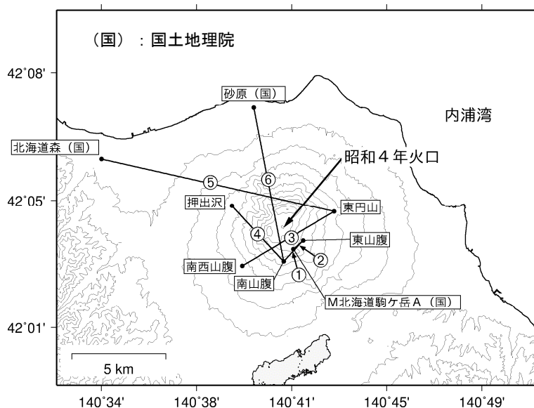
図7 北海道駒ヶ岳 GNSS連続観測による基線長変化(2001年4月～2024年1月)及び観測点配置図
