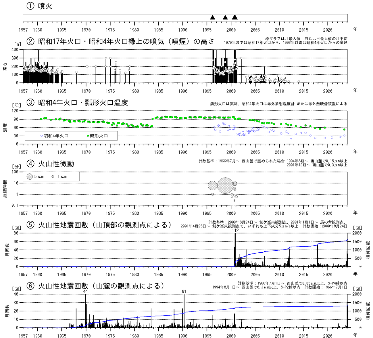
図1 北海道駒ヶ岳 火山活動経過図（1957年1月～2024年1月）
