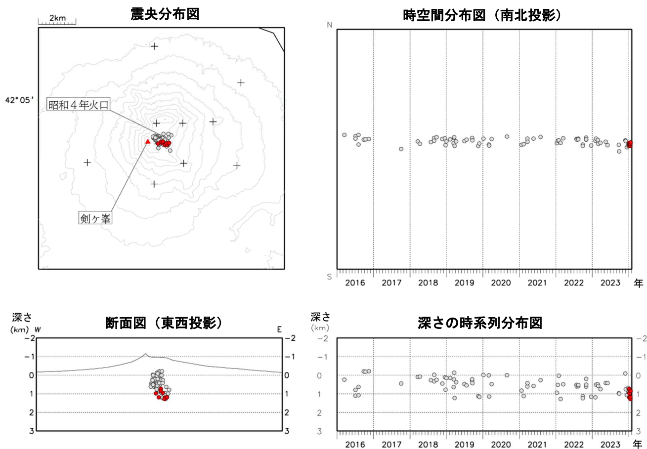
図6 北海道駒ヶ岳 火山性地震の震源分布（2016年1月～2024年1月）
