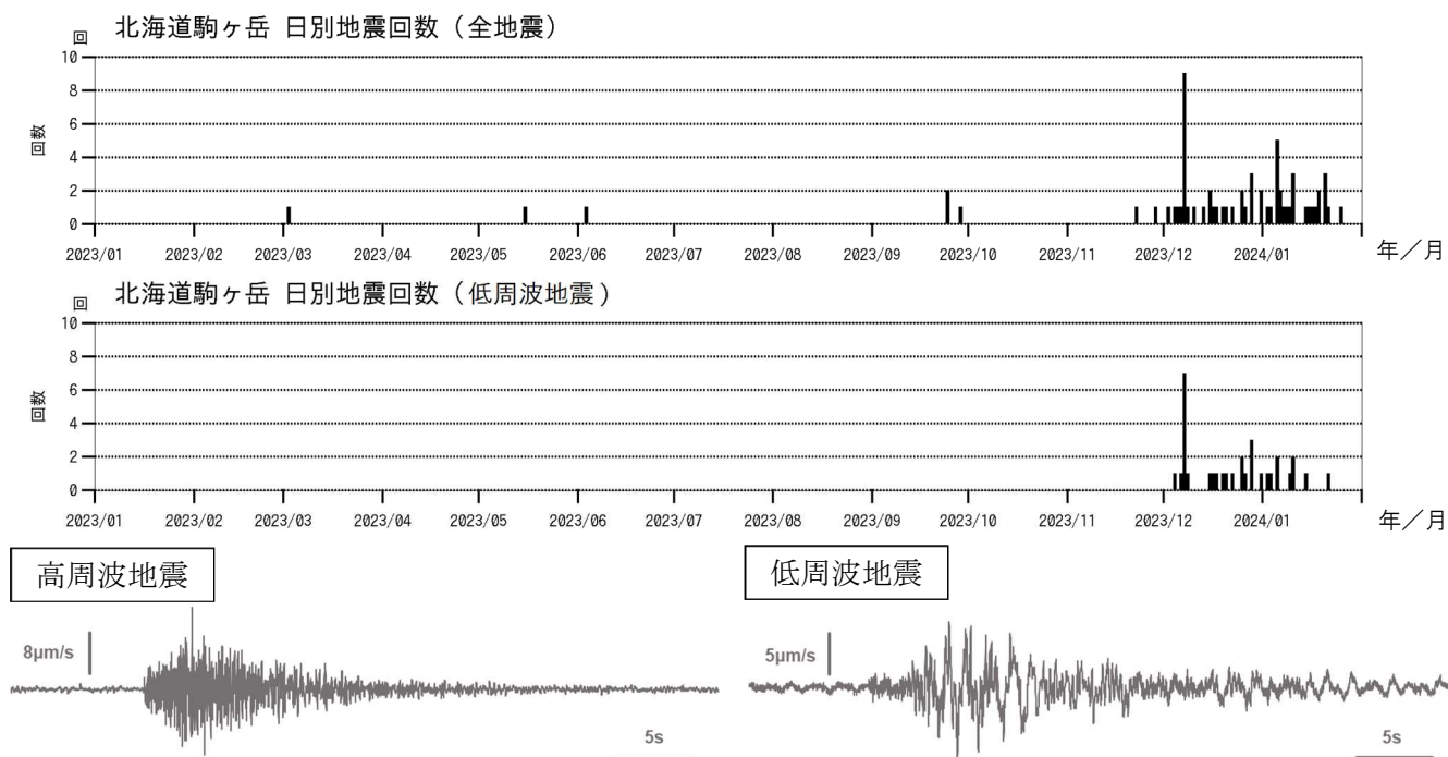
図5 北海道駒ヶ岳 日別地震回数（上段：全地震 下段：低周波地震 2023年1月～2024年1月）及び火山性地震の波形例（左下：高周波地震 右下：低周波地震）
