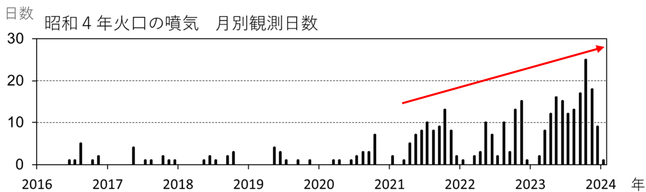
図4 北海道駒ヶ岳 昭和4年火口のごく弱い噴気を観測した日数（2016年1月～2024年1月）
