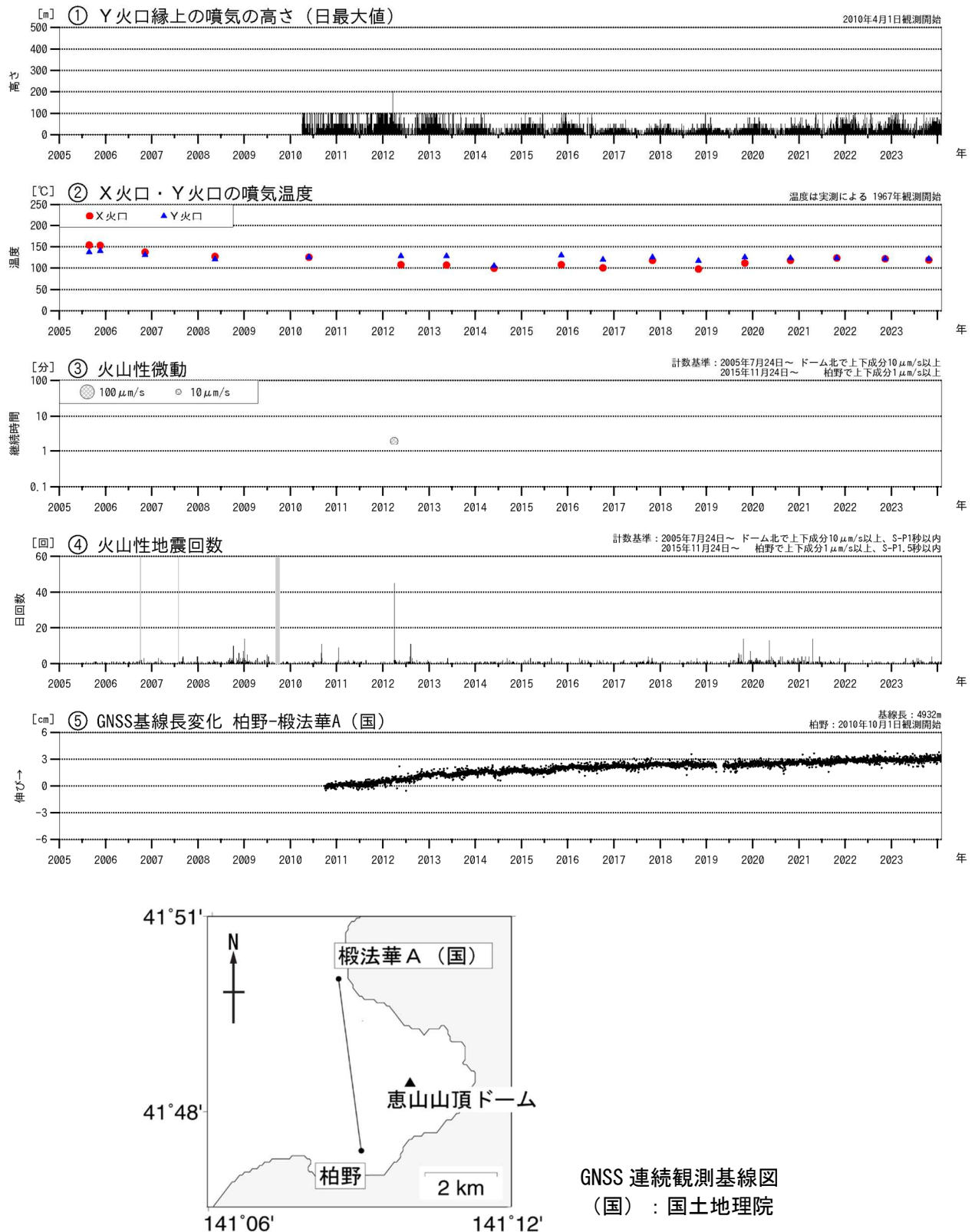
図2 恵山 火山活動経過図（2005年7月～2024年1月） ④の灰色部分は機器障害による欠測期間を示します。 ⑤のグラフは上図の基線に対応しています。 ⑤のグラフの空白部分は欠測を示します。
