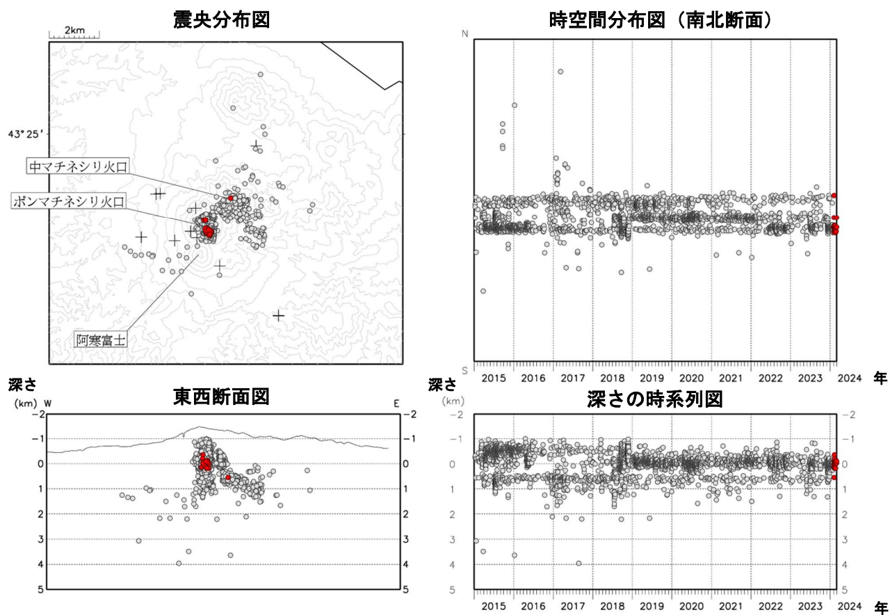
図4 雌阿寒岳 火山性地震の震源分布（2015年1月～2024年2月）
