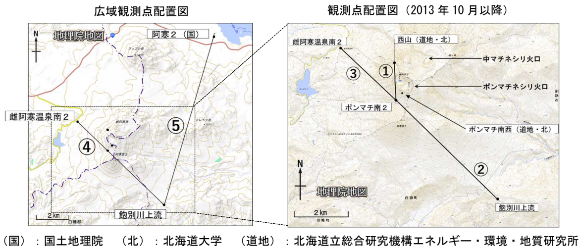
図5 雌阿寒岳 GNSS連続観測による基線長変化（2006年4月～2024年2月）及び観測点配置図
