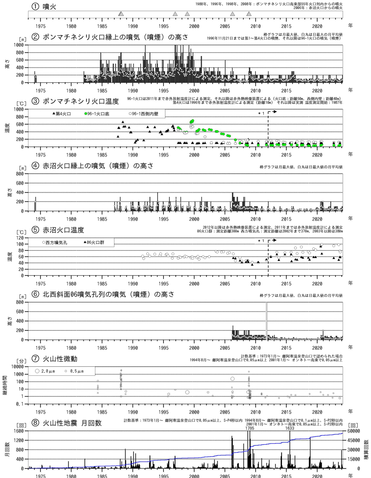
図1 雌阿寒岳 火山活動経過図（1973年1月～2024年2月）
