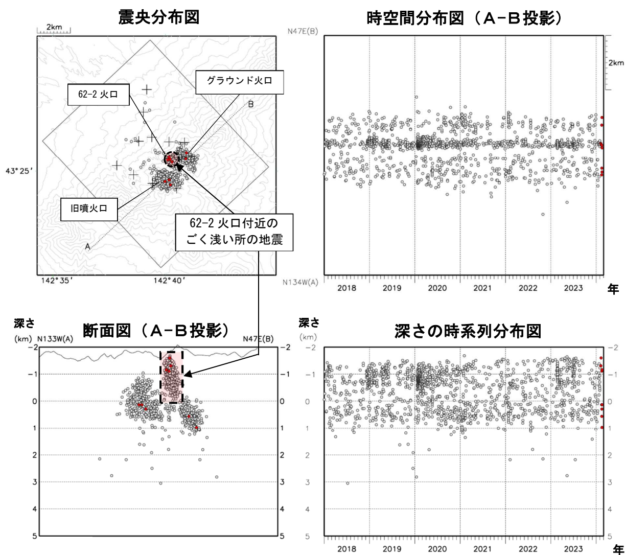
図4 十勝岳 火山性地震の震源分布（2018年1月～2024年2月）
