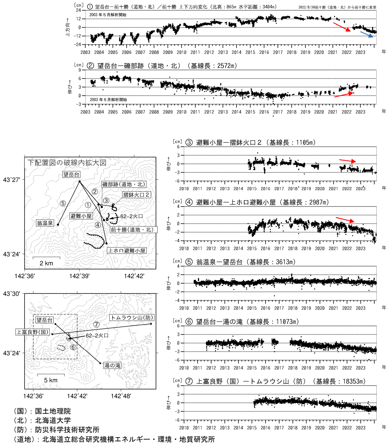
図5 十勝岳 GNSS連続観測による上下方向変化及び基線長変化（2003年5月～2024年2月）及び観測点配置図
