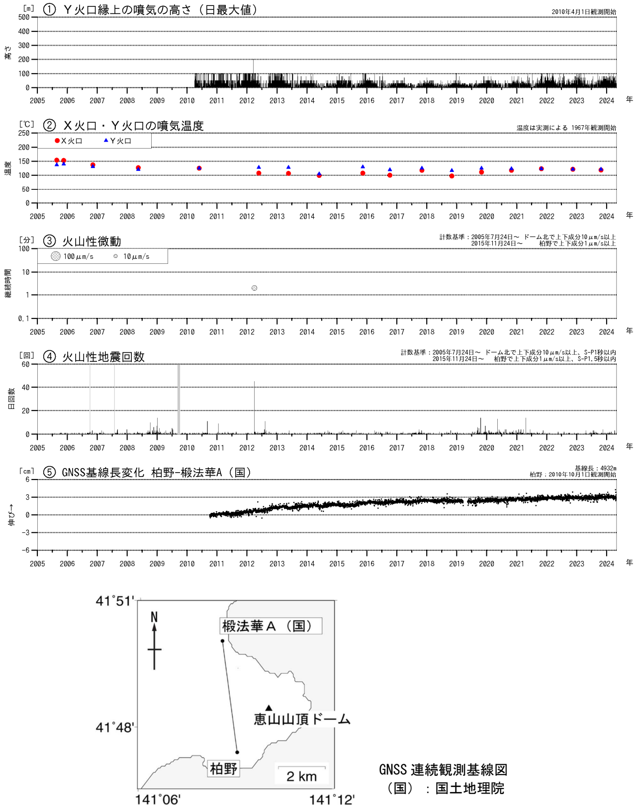
図2 恵山 火山活動経過図（2005年7月～2024年4月） ④の灰色部分は機器障害による欠測期間を示します。 ⑤のグラフは上図の基線に対応しています。 ⑤のグラフの空白部分は欠測を示します。
