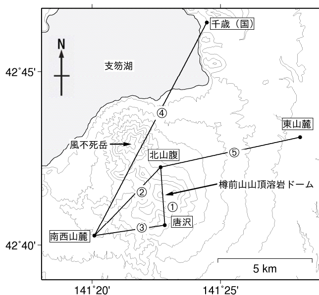
図4 樽前山 GNSS連続観測による基線長変化（2005年1月～2024年5月）及び観測点配置図
