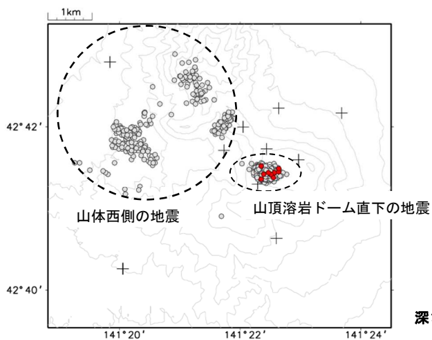
震央分布図
