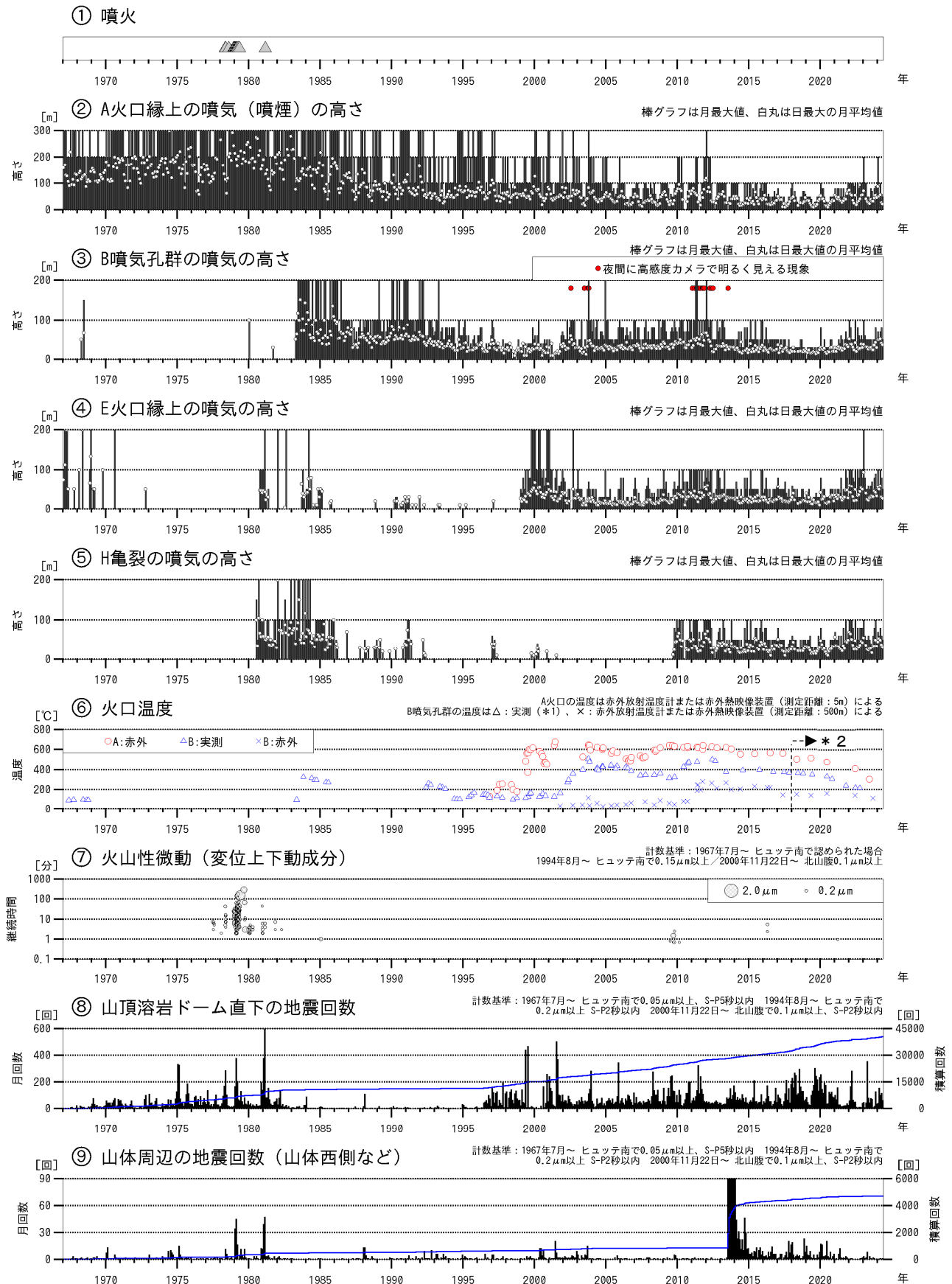
図2 樽前山 火山活動経過図（1967年1月～2024年5月）
