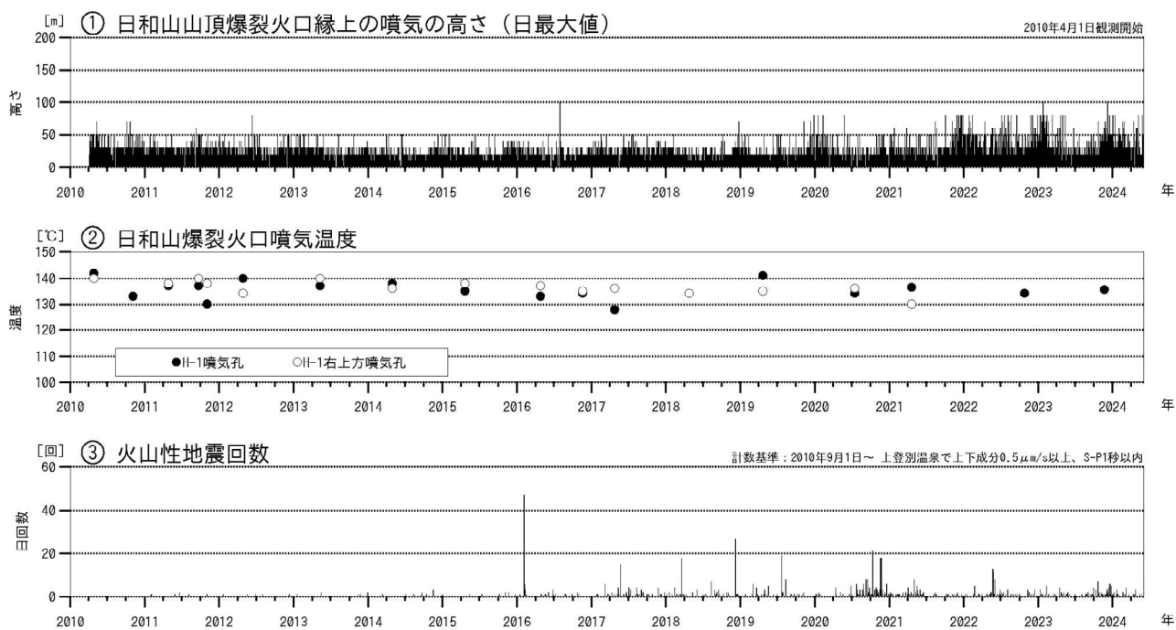
図2 倶多楽 火山活動経過図（2010年1月～2024年5月）
