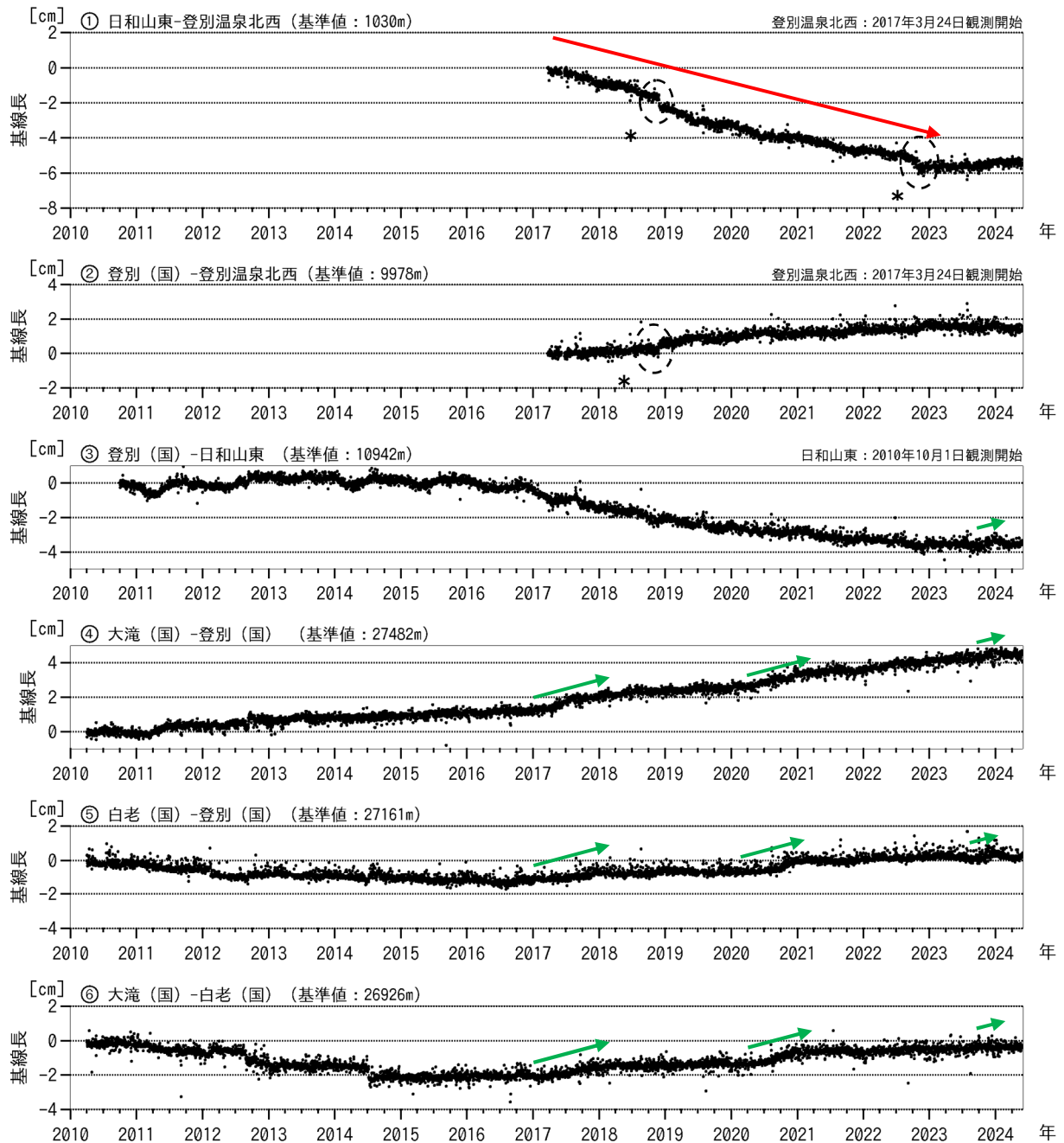
図3 倶多楽 GNSS連続観測による基線長変化（2010年4月～2024年5月）
