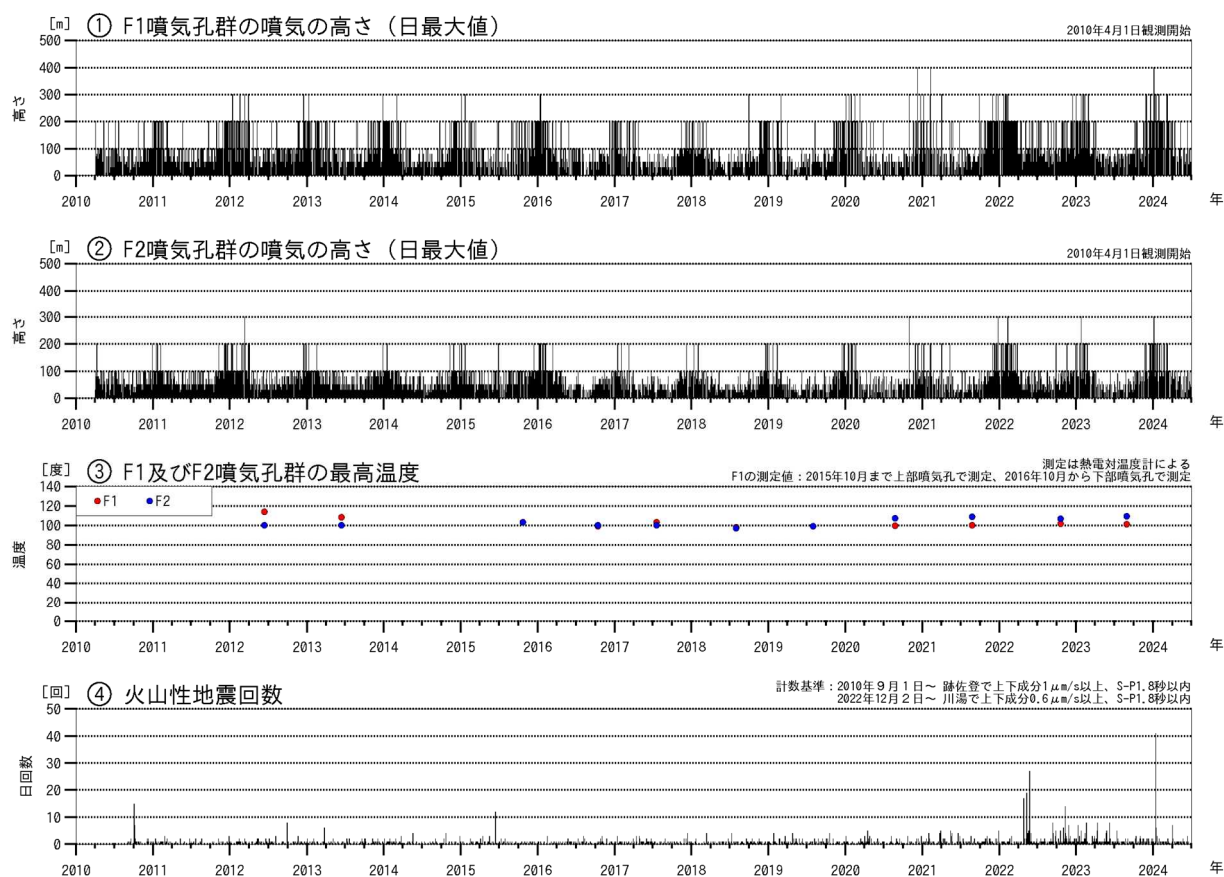
図1 アトサヌプリ 火山活動経過図（2010年4月～2024年6月）
