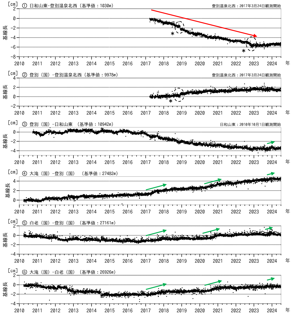
図3 倶多楽 GNSS連続観測による基線長変化（2010年4月～2024年6月）
