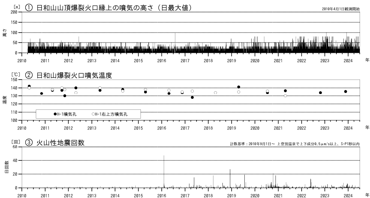
図2 倶多楽 火山活動経過図（2010年1月～2024年6月）
