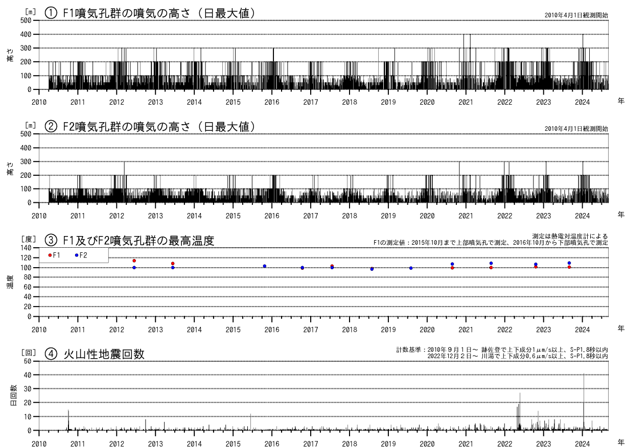
図1 アトサヌプリ 火山活動経過図（2010年4月～2024年8月）
