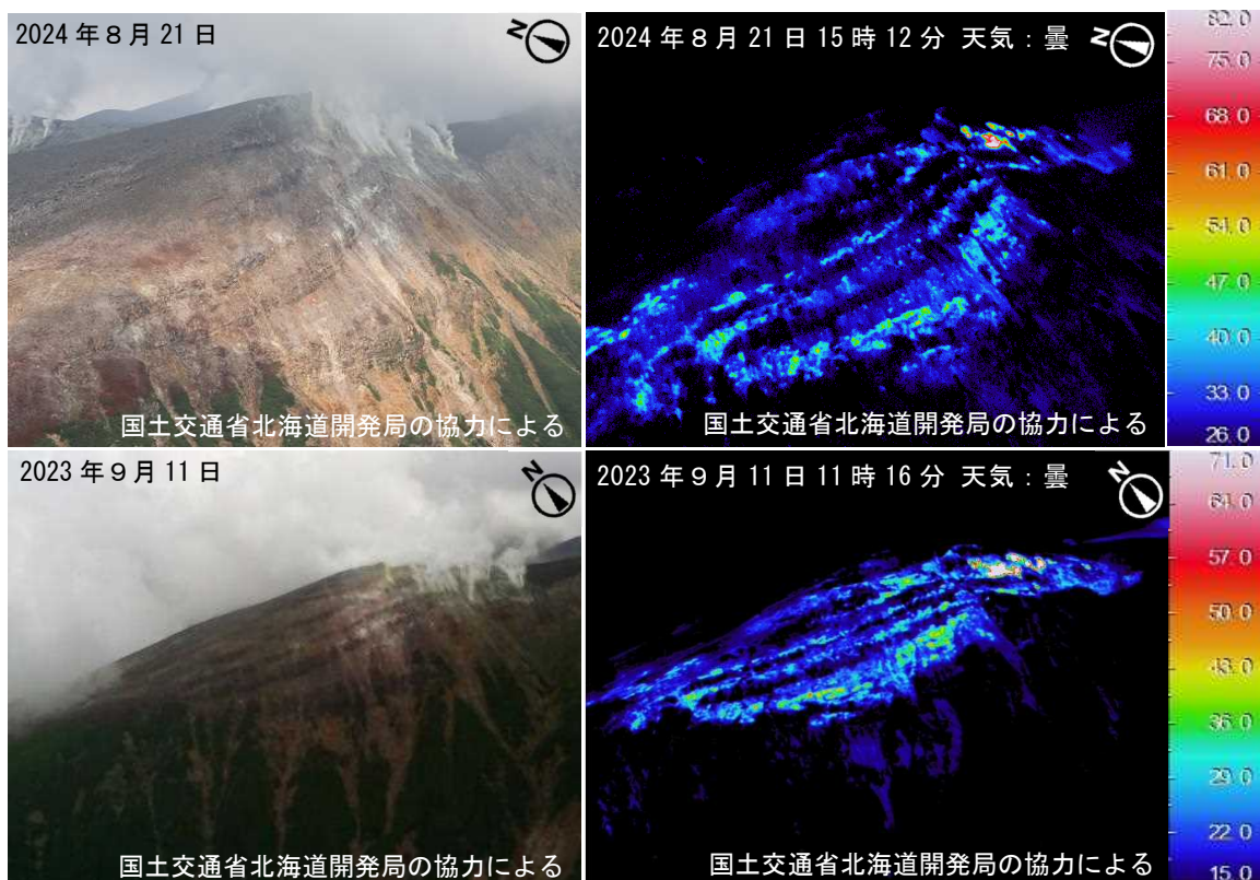
図6 十勝岳 赤外熱映像装置による振子沢噴気孔群の地表面温度分布
