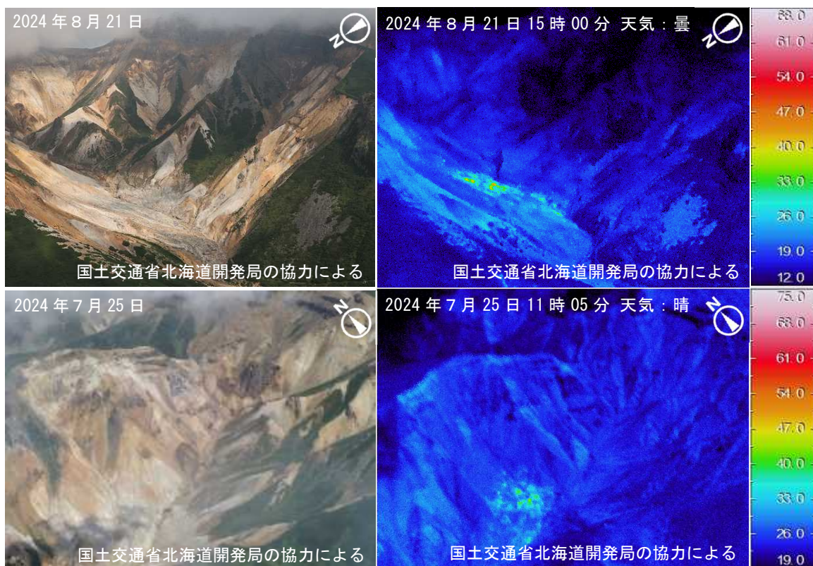
図7 十勝岳 赤外熱映像装置による旧噴火口の地表面温度分布
