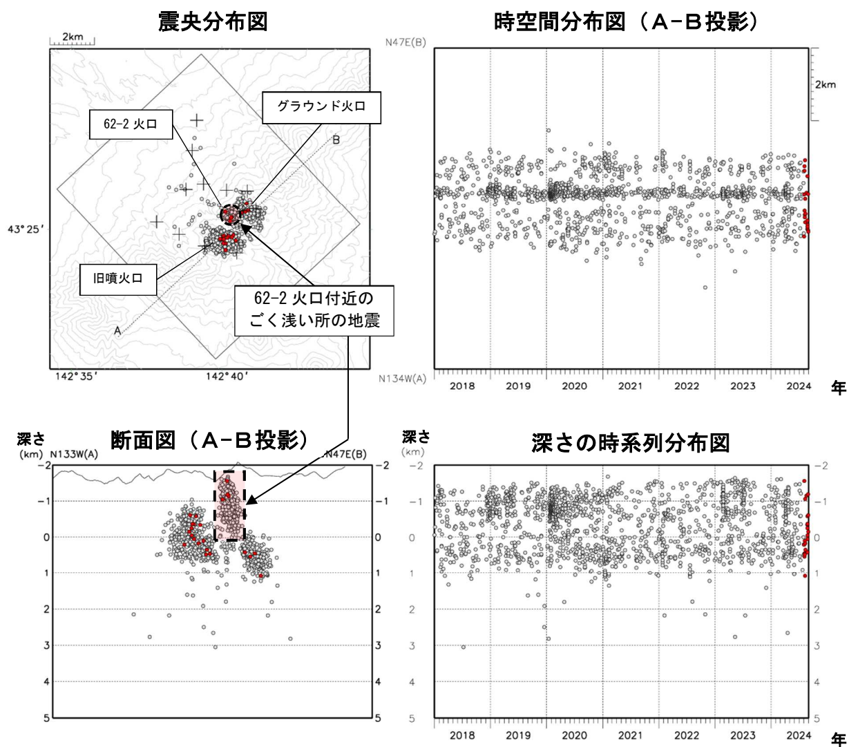
図8 十勝岳 火山性地震の震源分布（2018年1月～2024年8月）
