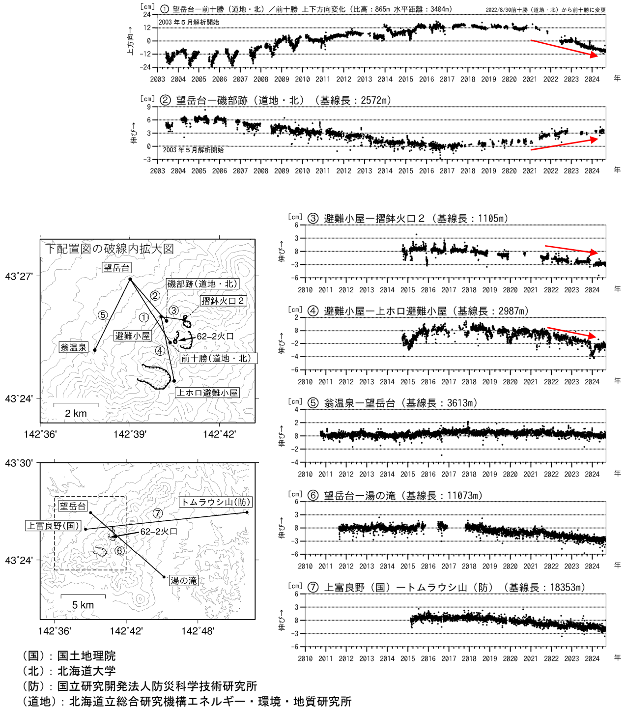
図9 十勝岳 GNSS連続観測による上下方向変化及び基線長変化（2003年5月～2024年8月）及び観測点配置図
