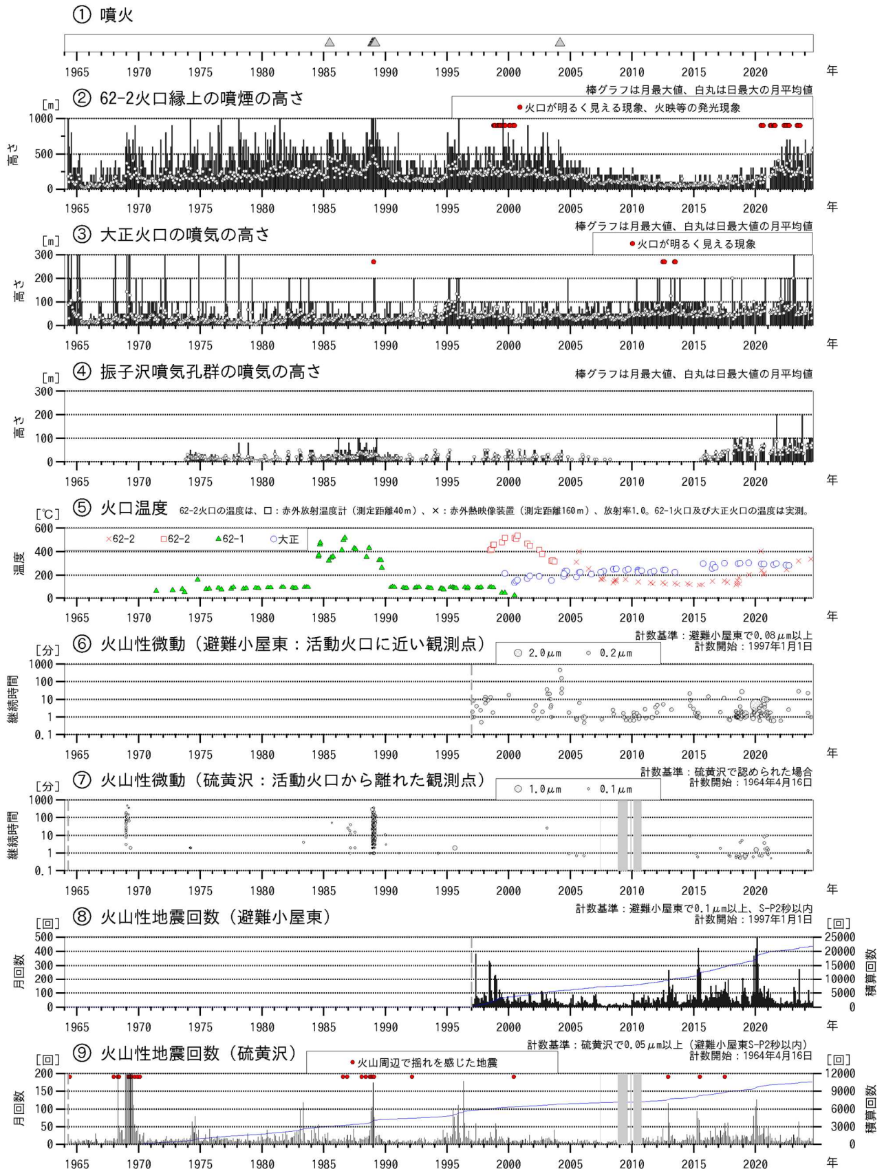
図1 十勝岳 火山活動経過図（1964年1月～2024年8月）
