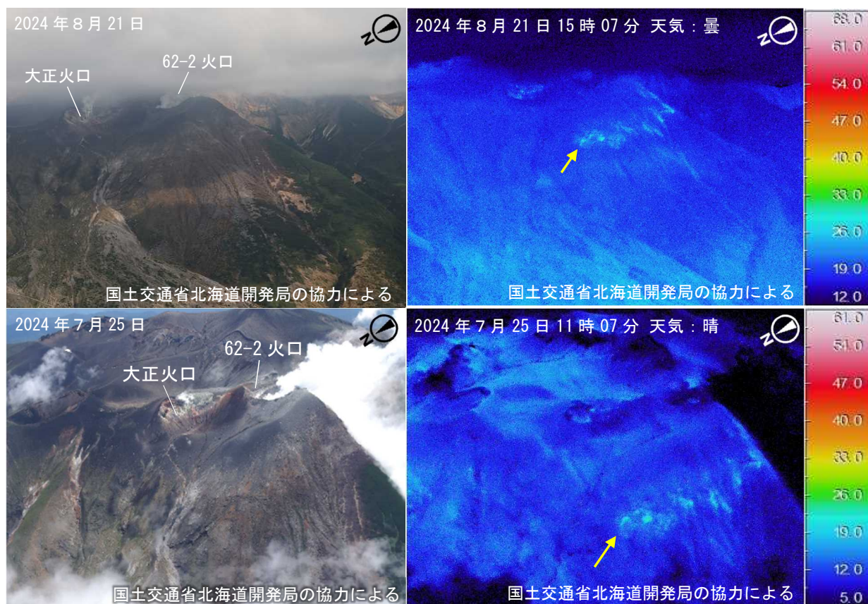
図5 十勝岳 赤外熱映像装置による前十勝北西側斜面の地表面温度分布
