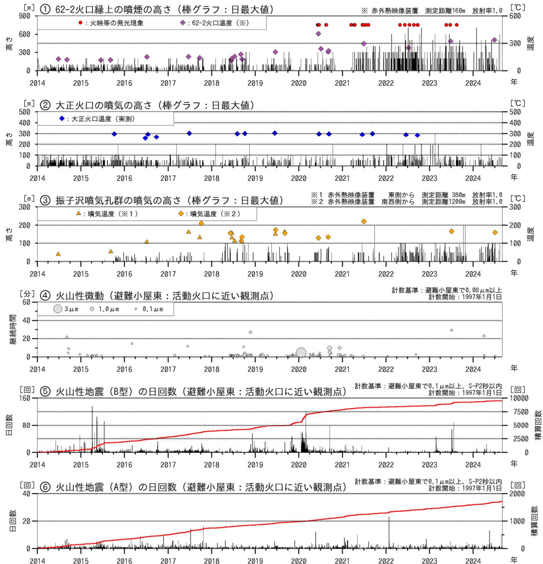
図2 十勝岳 火山活動経過図（2014年1月～2024年8月）
