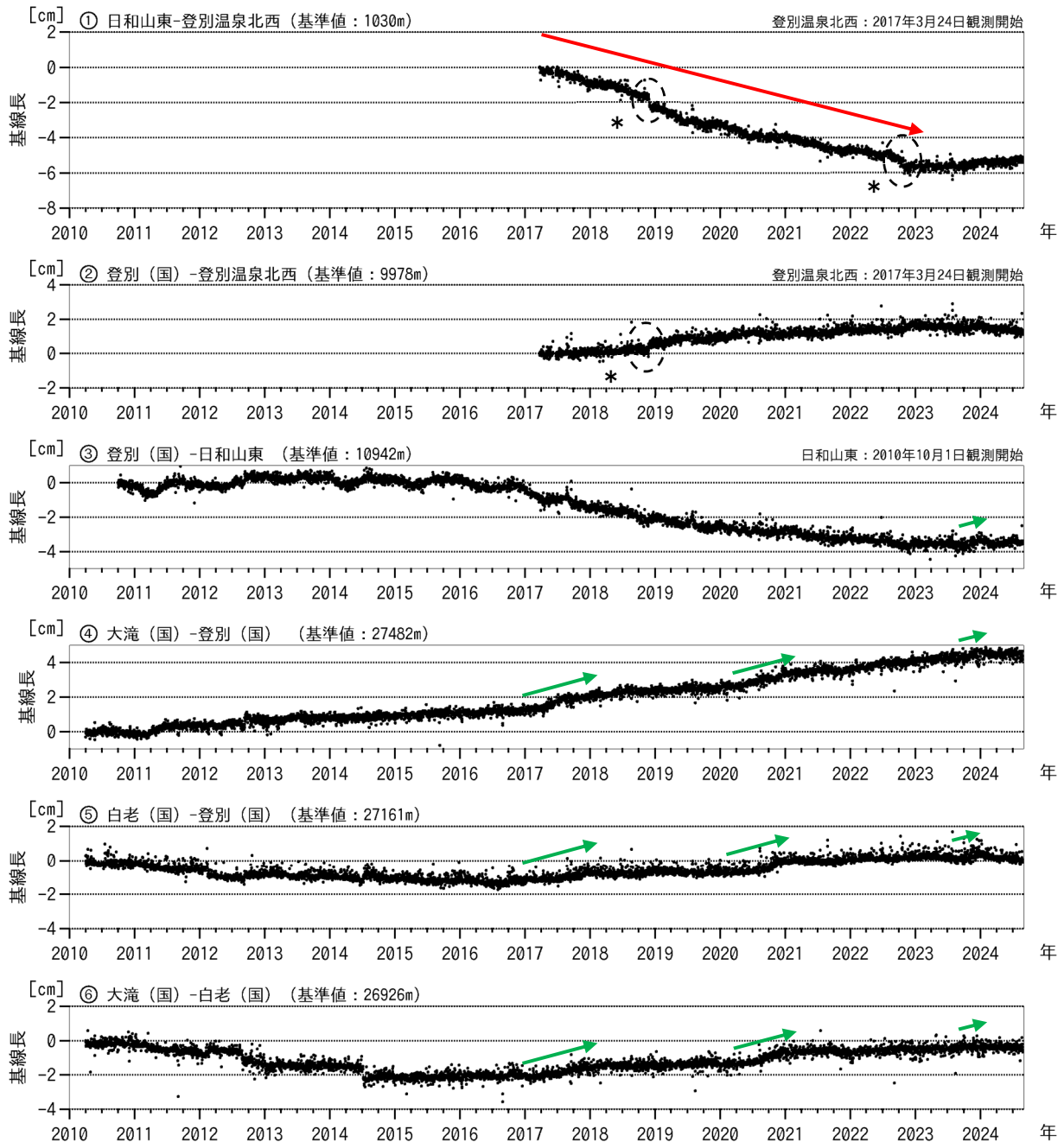
図3 倶多楽 GNSS連続観測による基線長変化（2010年4月～2024年8月）
