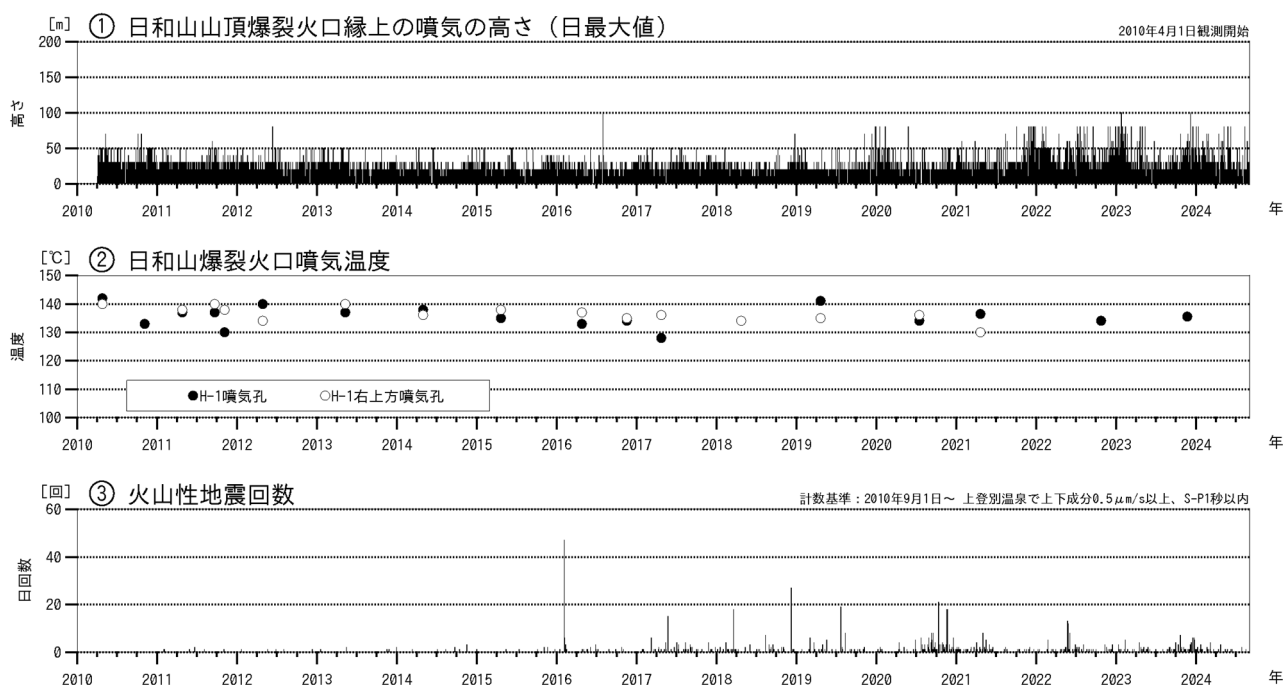
図2 倶多楽 火山活動経過図（2010年1月～2024年8月）
