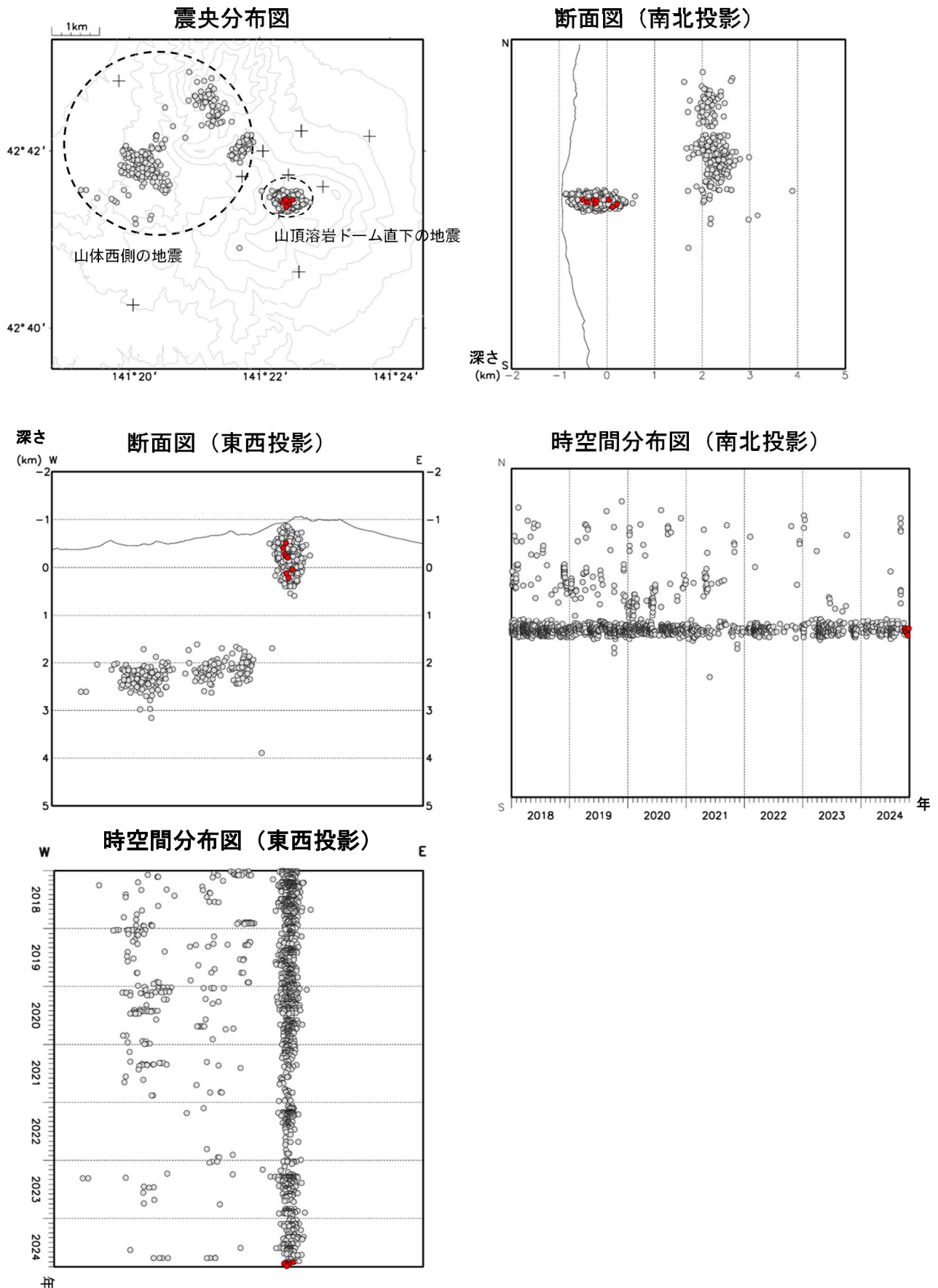
図5 樽前山 火山性地震の震源分布（2018年1月～2024年10月）
