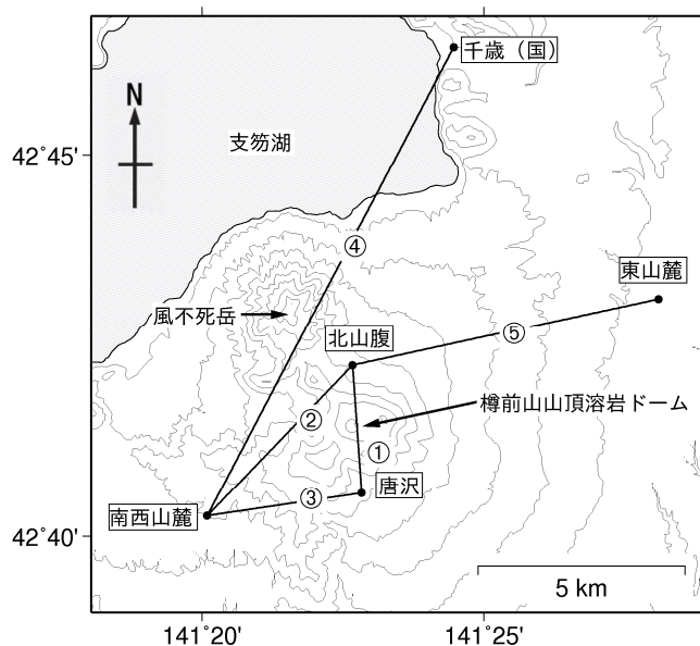
図6 樽前山 GNSS連続観測による基線長変化（2005年1月～2024年10月）及び観測点配置図 グラフ①～⑤は観測点配置図の基線①～⑤に対応しています。 グラフ中の空白部分は欠測を示しています。 ②～④の楕円内の変動（* 1）は2014年7月8日に発生した胆振地方中東部の地震によるものです。
