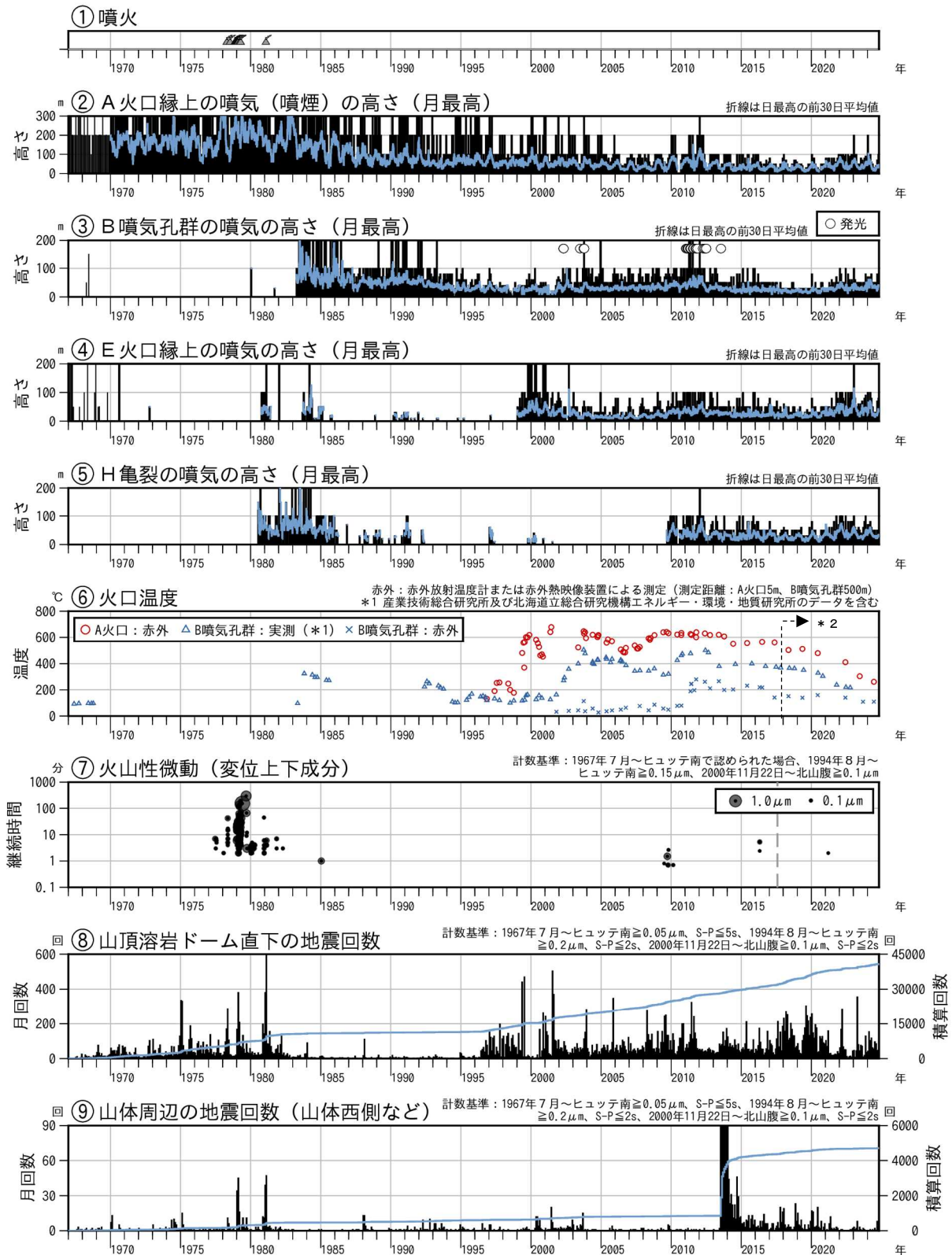
図4 樽前山 火山活動経過図（1967年1月～2024年10月）
