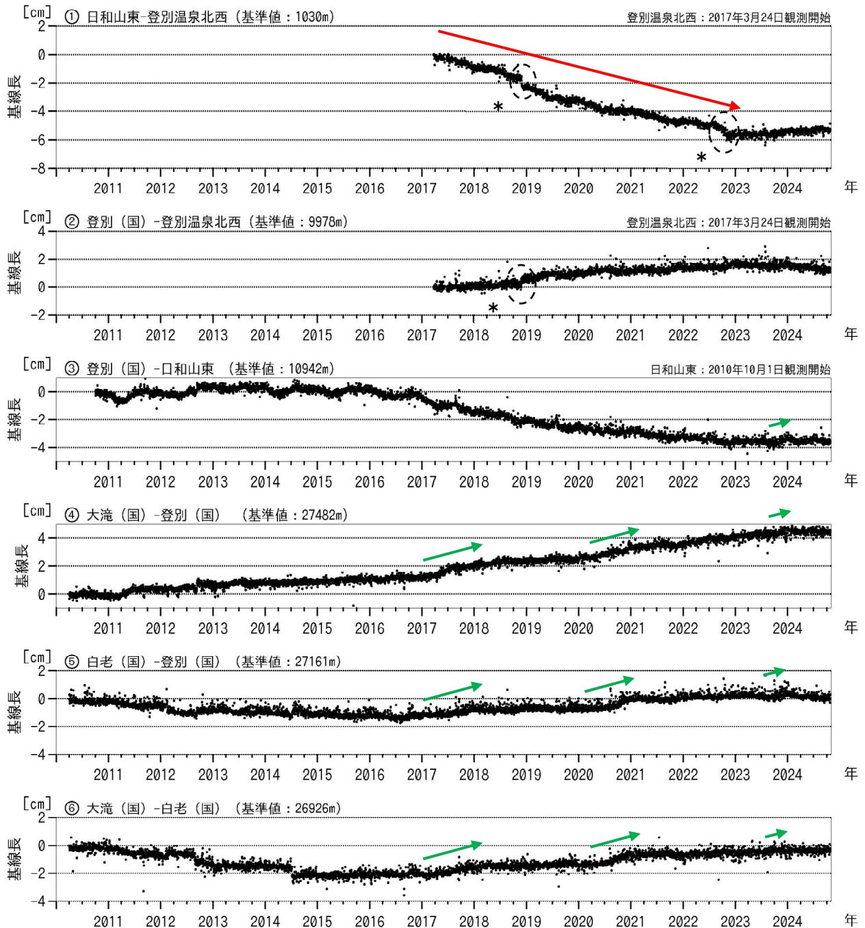
図5 倶多楽 GNSS連続観測による基線長変化（2010年4月～2024年10月）
