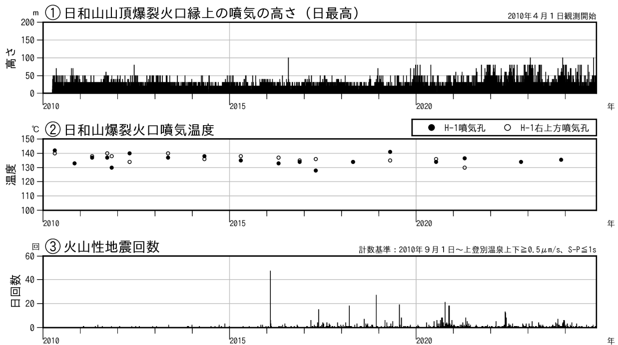
図2 倶多楽 火山活動経過図（2010年1月～2024年10月）
