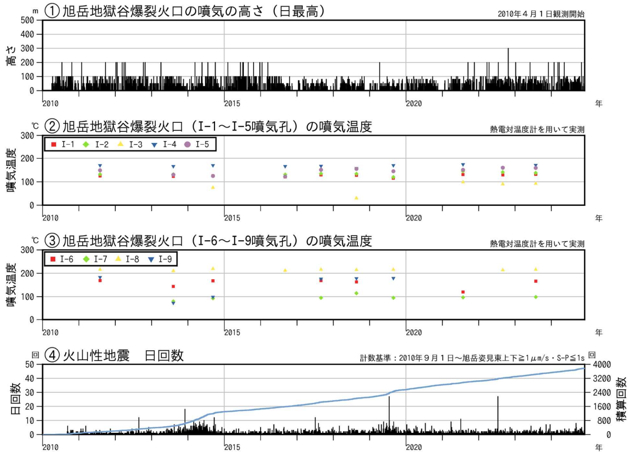
図2 大雪山 火山活動経過図（2010年4月～2024年11月）
