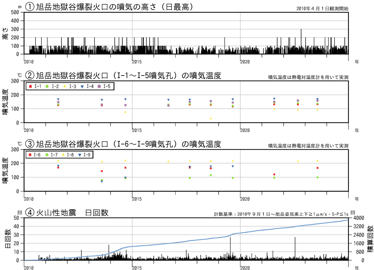
図2 大雪山 火山活動経過図 (2010年4月～2024年12月)
