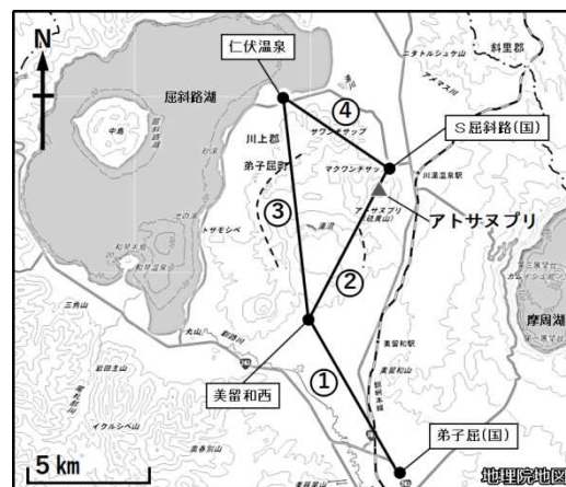
図4 アトサヌプリ GNSS連続観測による基線長変化（2010年10月～2025年1月）及び観測点配置図
