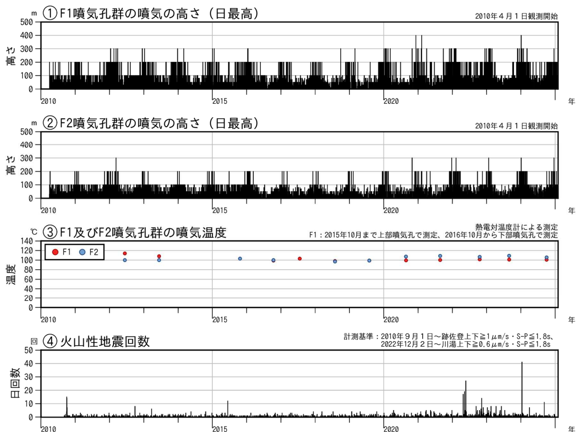
図1 アトサヌプリ 火山活動経過図（2010年4月～2025年1月）
