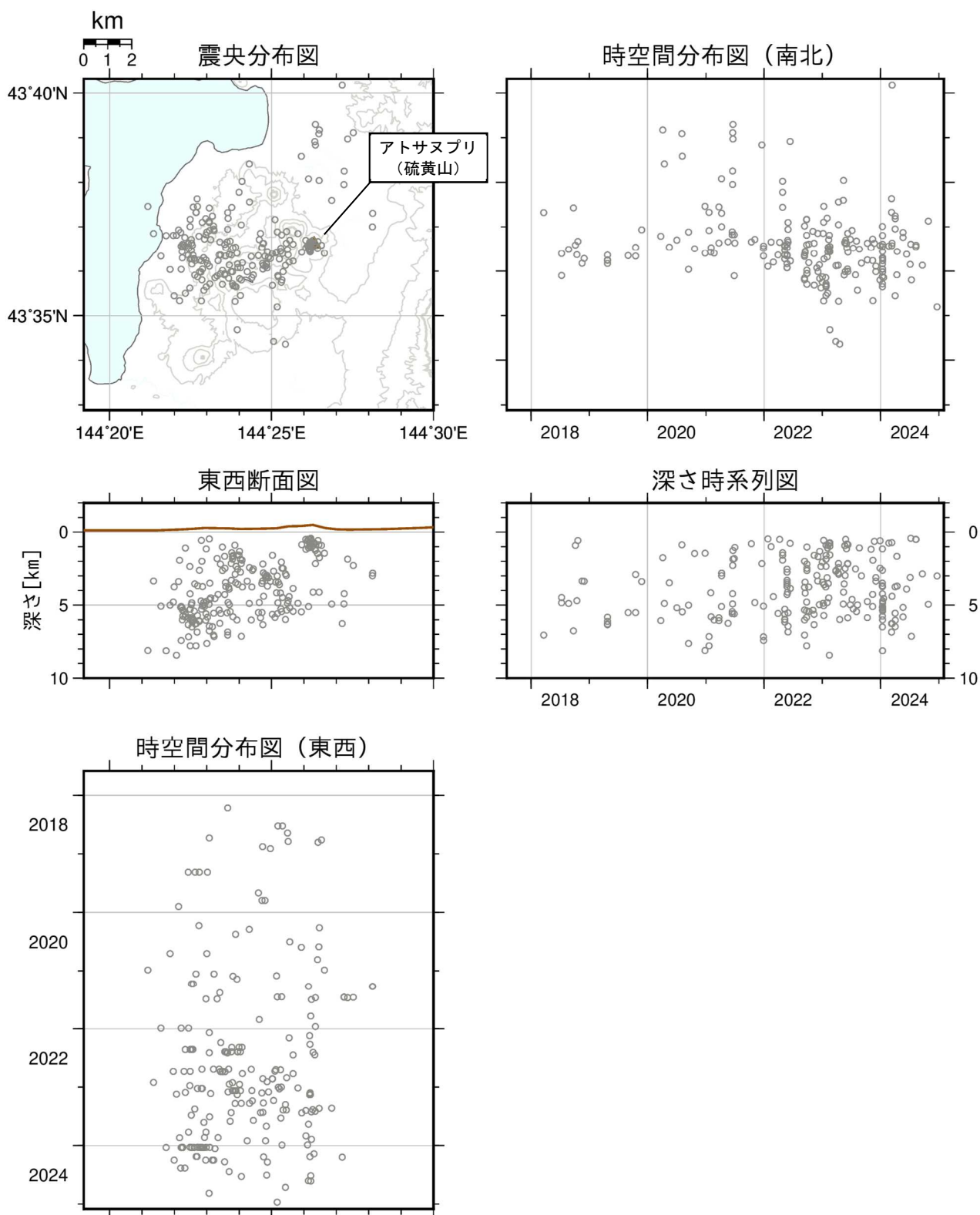
図3 アトサヌプリ 火山性地震の震源分布（2017年8月～2025年1月）
