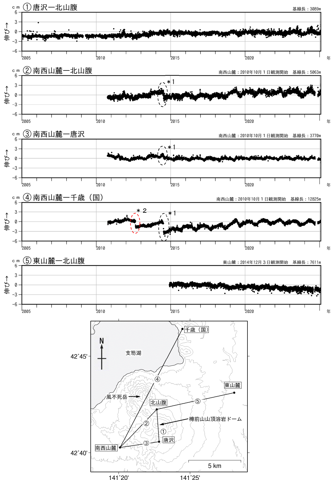
図4 樽前山 GNSS連続観測による基線長変化（2005年1月～2025年1月）及び観測点配置図
