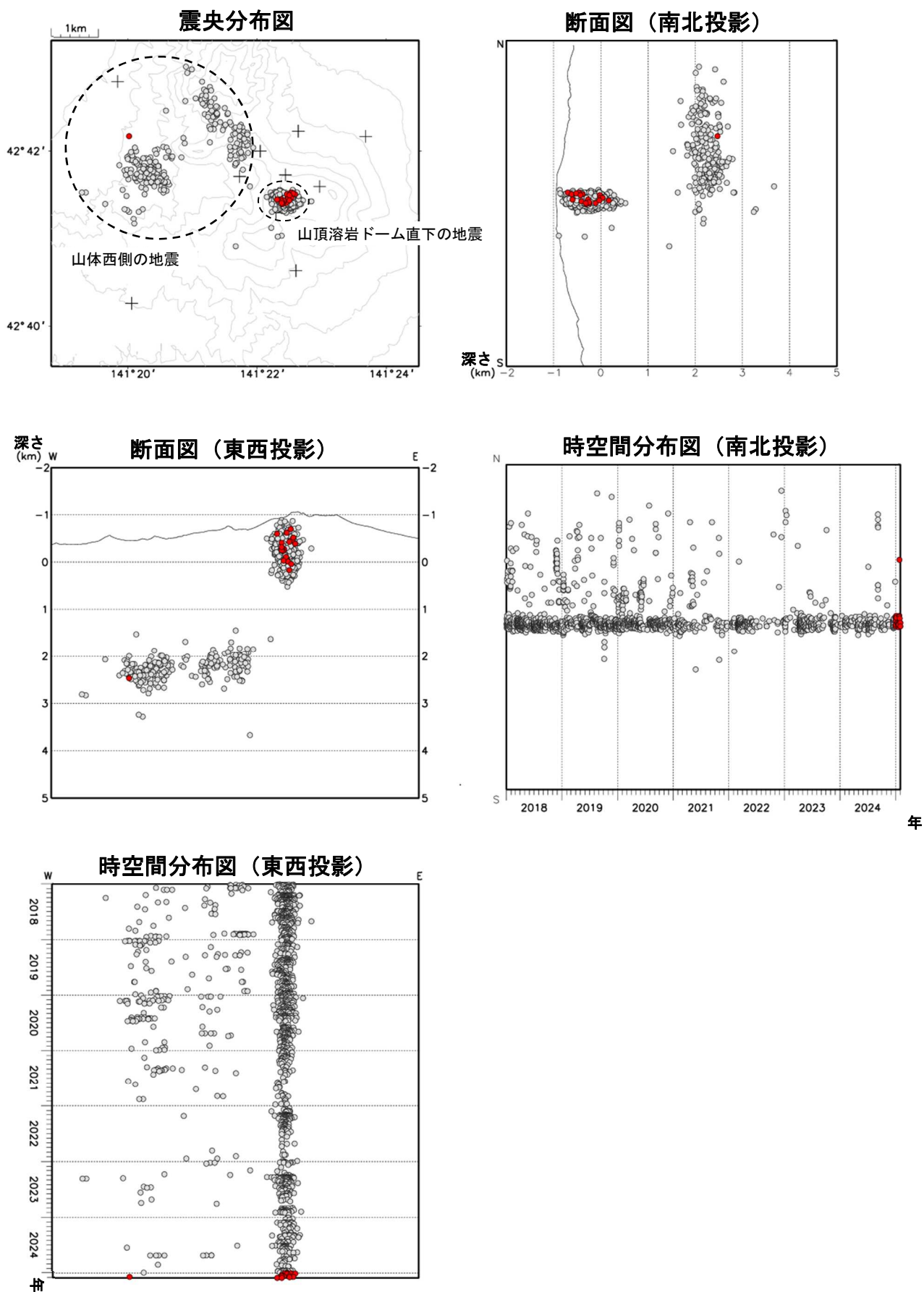
図3 樽前山 火山性地震の震源分布（2018年1月～2025年1月）
