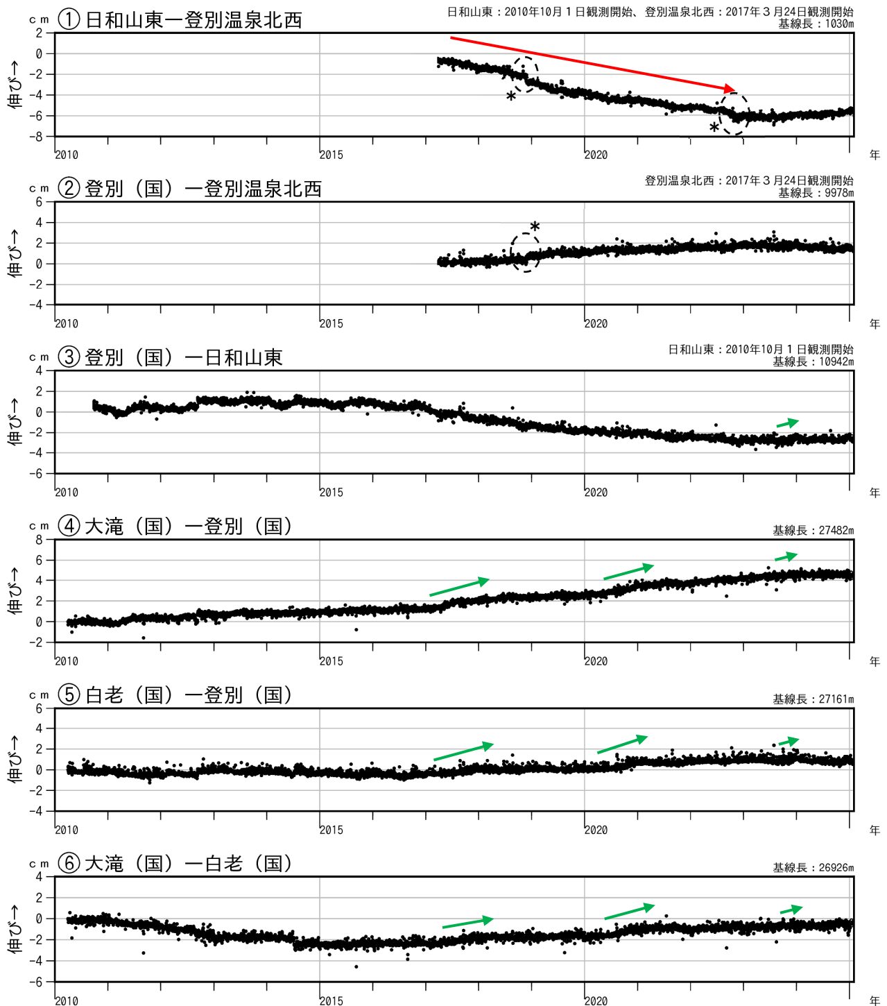
図3 倶多楽 GNSS連続観測による基線長変化（2010年4月～2025年1月）
