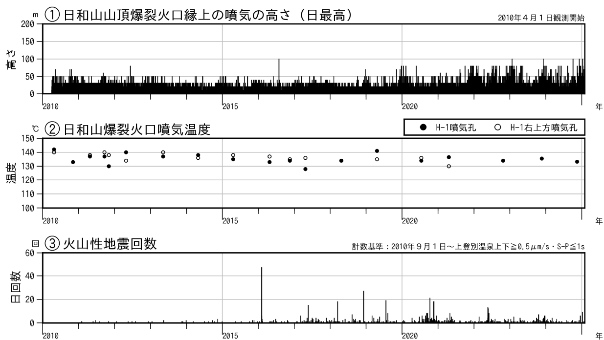
図 2 倶多楽 火山活動経過図（2010年 1 月～2025年 1 月）
