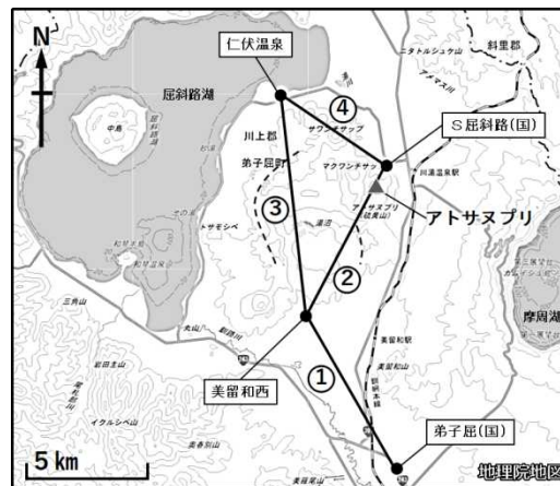
図4 アトサヌプリ GNSS連続観測による基線長変化（2010年10月～2025年3月）及び観測点配置図 冬季に凍上や積雪の影響によると考えられる変動がみられる基線があります。
