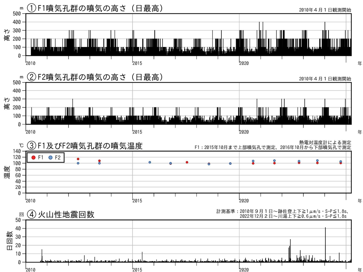
図 1 アトサヌプリ 火山活動経過図（2010年 4 月～2025年 3 月）
