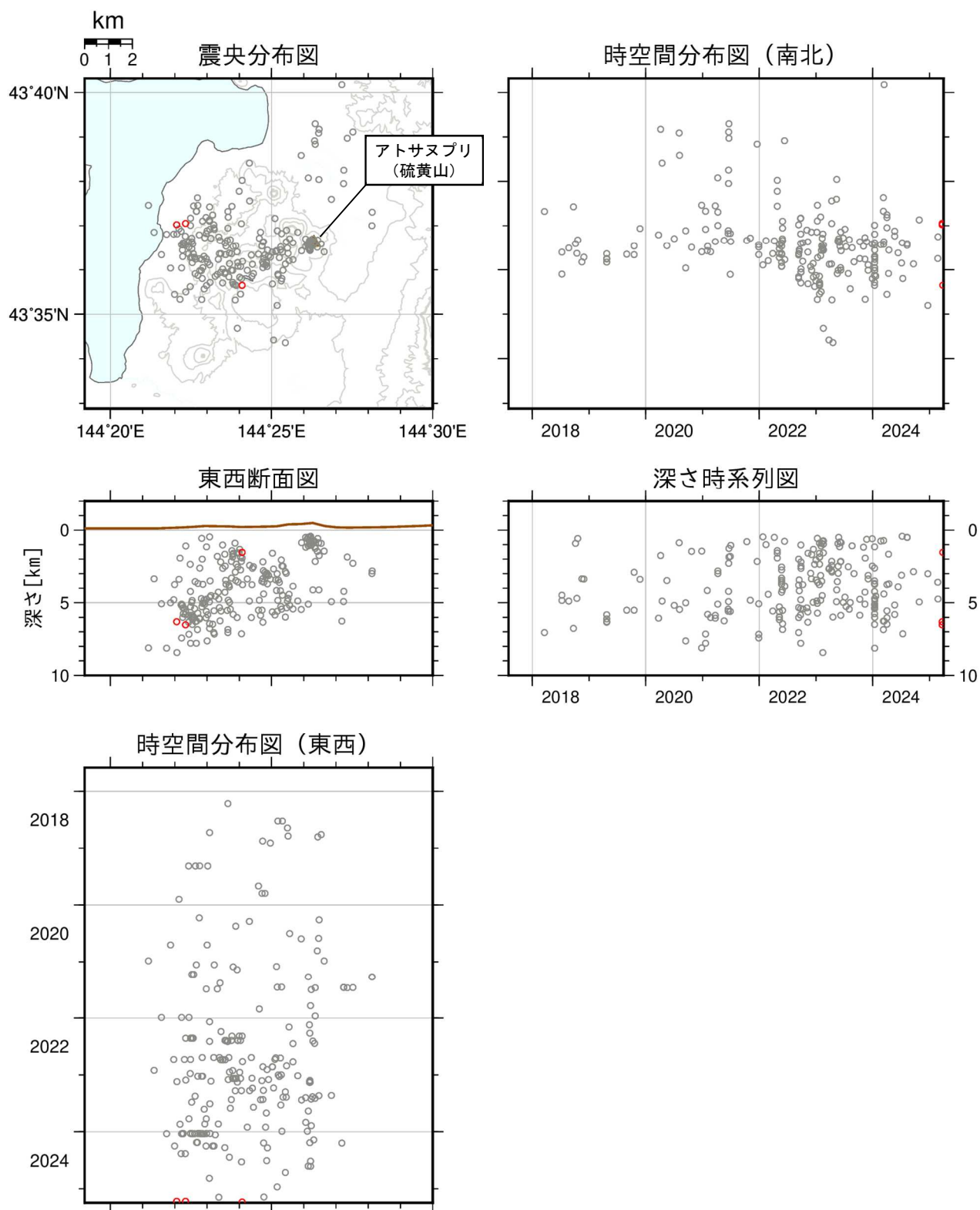
図3 アトサヌプリ 火山性地震の震源分布（2017年8月～2025年3月） ○：2017年8月～2025年2月の震源 ○：2025年3月の震源
