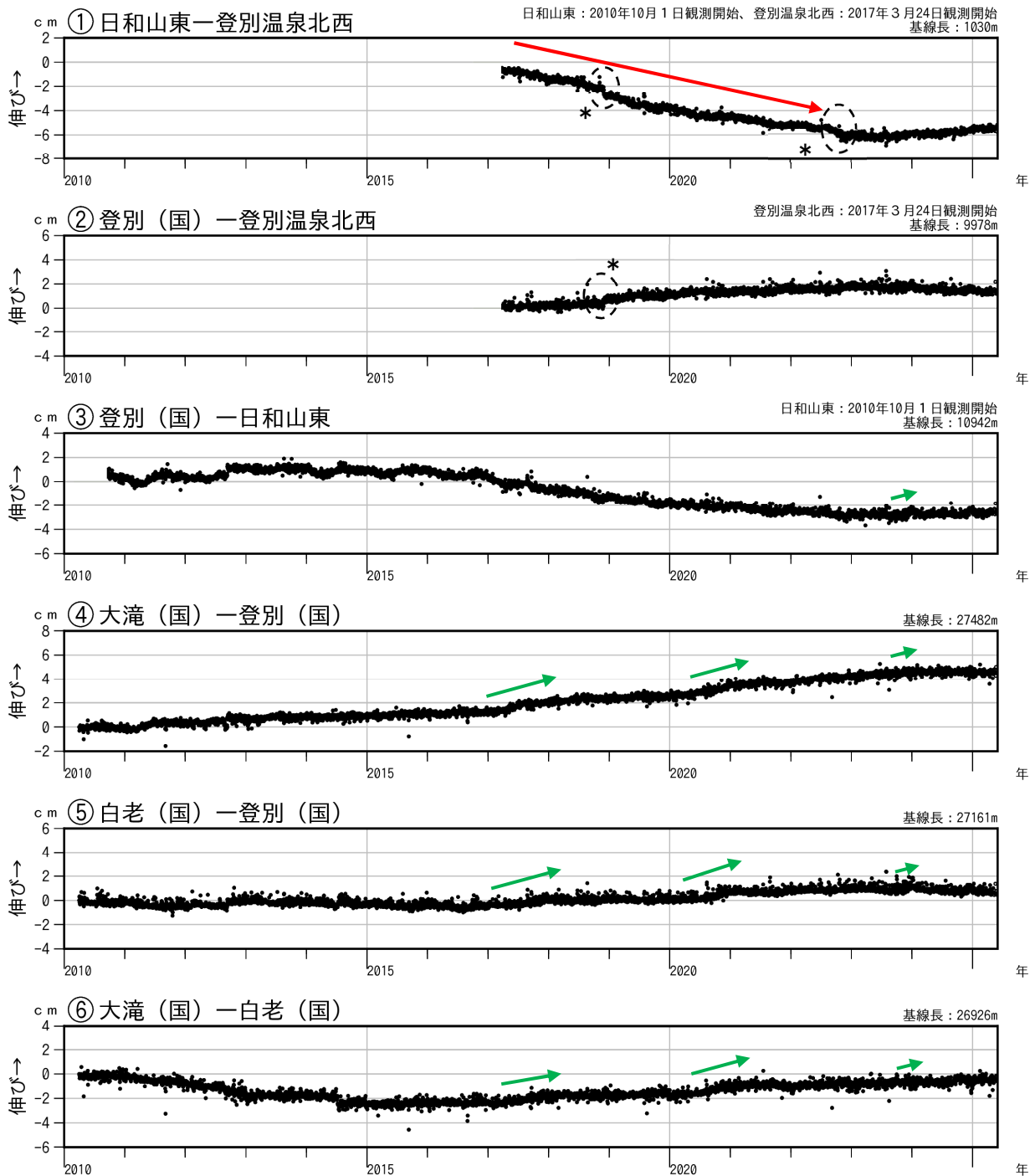
図3 倶多楽 GNSS連続観測による基線長変化（2010年4月～2025年5月）
