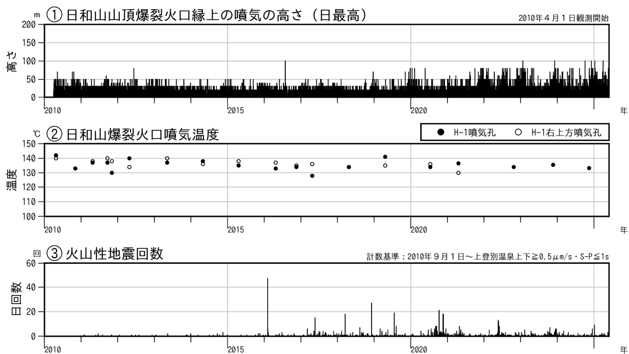
図 2 倶多楽 火山活動経過図（2010年 1 月～2025年 5 月）
