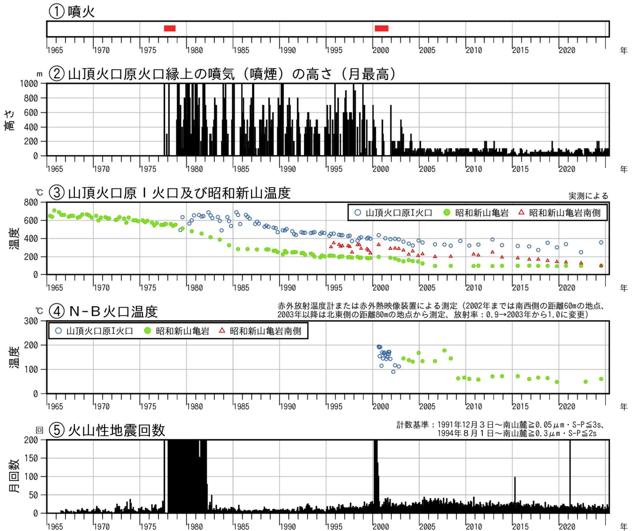
図1 有珠山 火山活動経過図（1965年1月～2025年5月）
