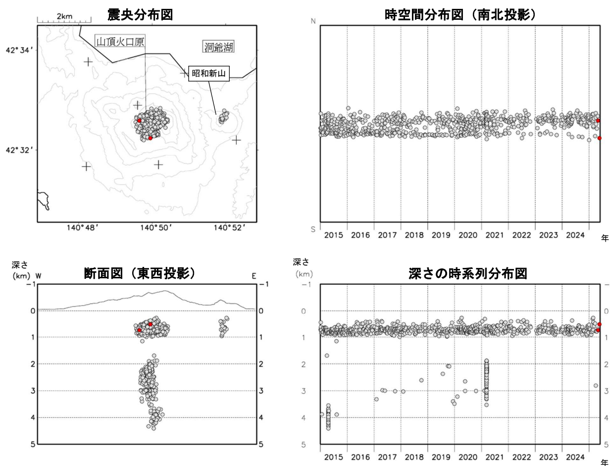
図3 有珠山 火山性地震の震源分布（2015年1月～2025年5月）
