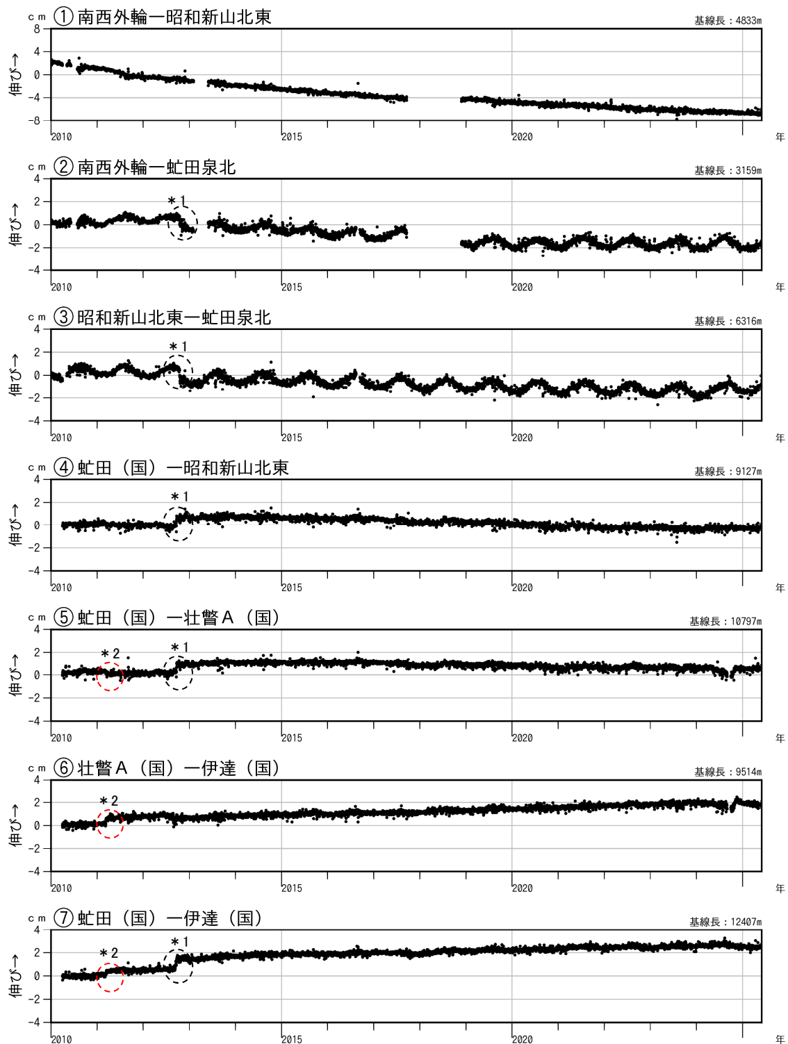
図4 有珠山 GNSS連続観測による基線長変化（2010年1月～2025年5月）
