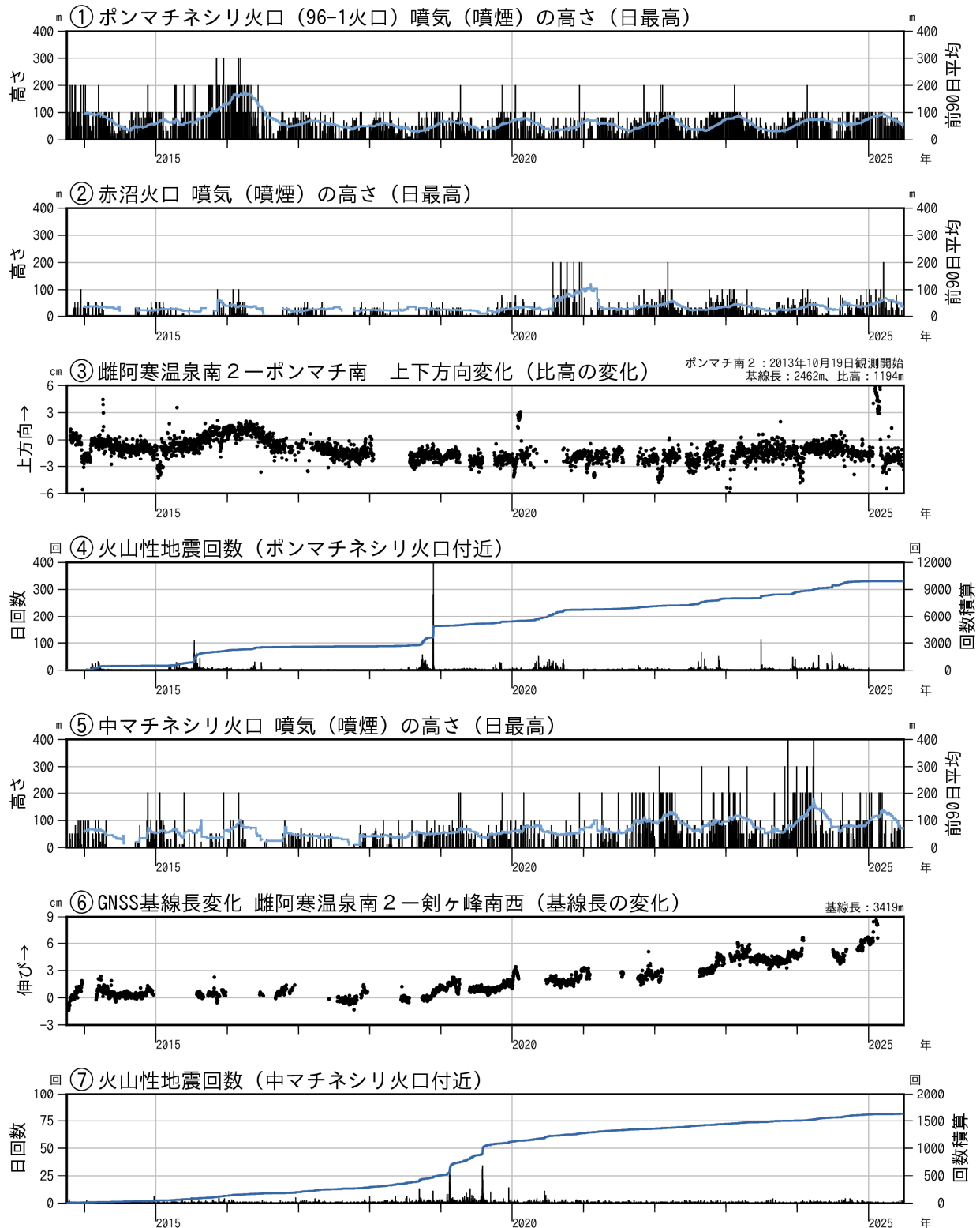
図5 雌阿寒岳 火口別の活動経過図（2013年10月～2025年6月）
