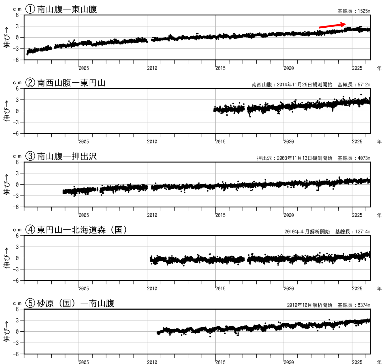
図4 北海道駒ヶ岳 GNSS連続観測による基線長変化（2001年4月～2026年4月）
