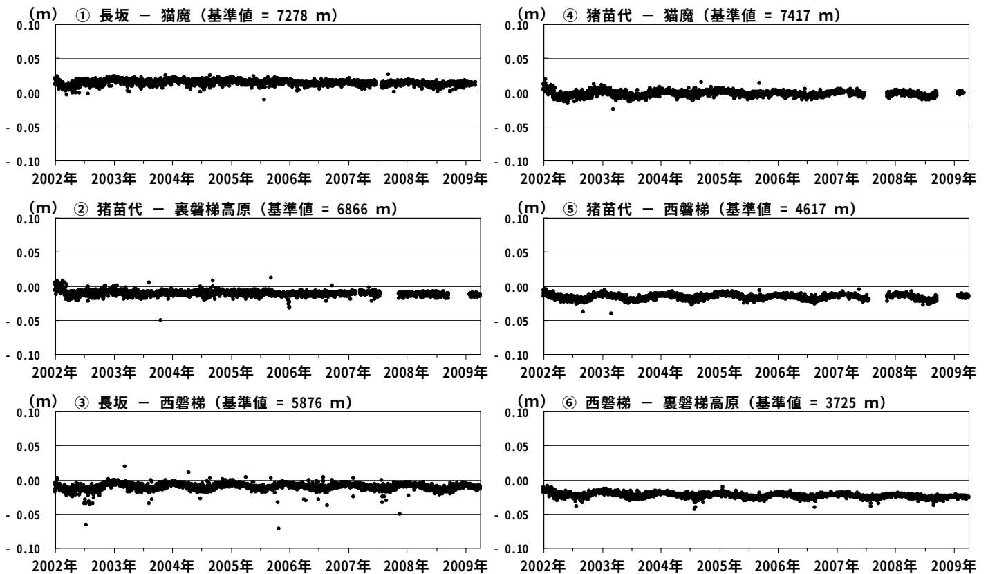
図6 磐梯山 GPS 基線長変化図（2002 年 1 月～2009 年 3 月）
