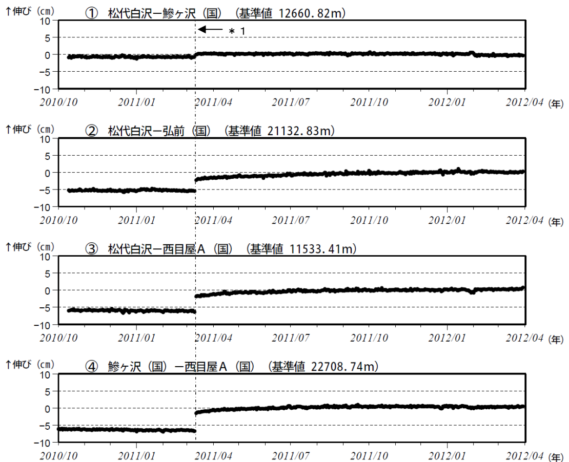
図 5※ 岩木山 GPS 基線長変化図（2010 年 10 月～2012 年 3 月）
