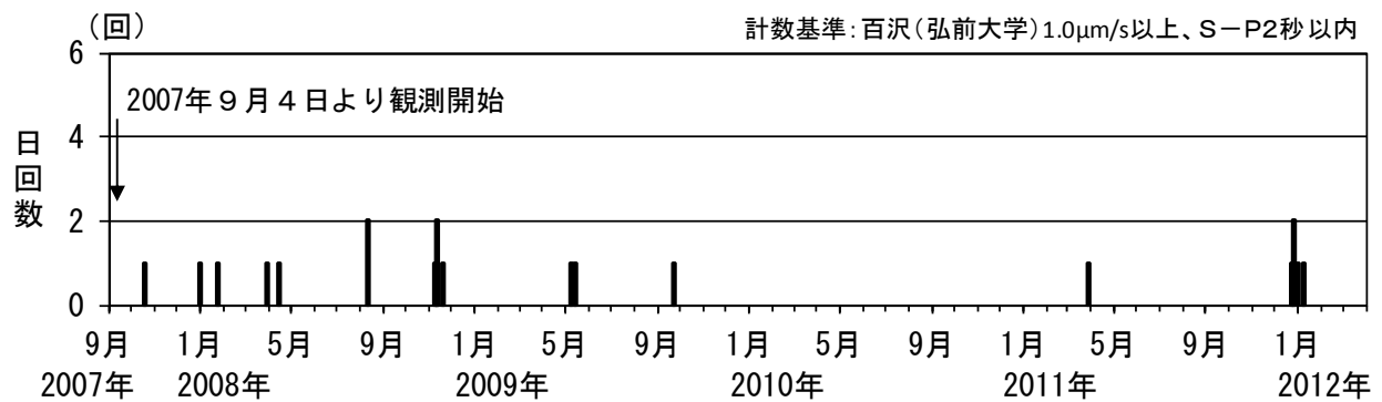
図3※ 岩木山 日別地震回数（2007年9月～2012年3月） 弘前大学からのデータ提供により、2007年9月4日から観測を開始しています。
