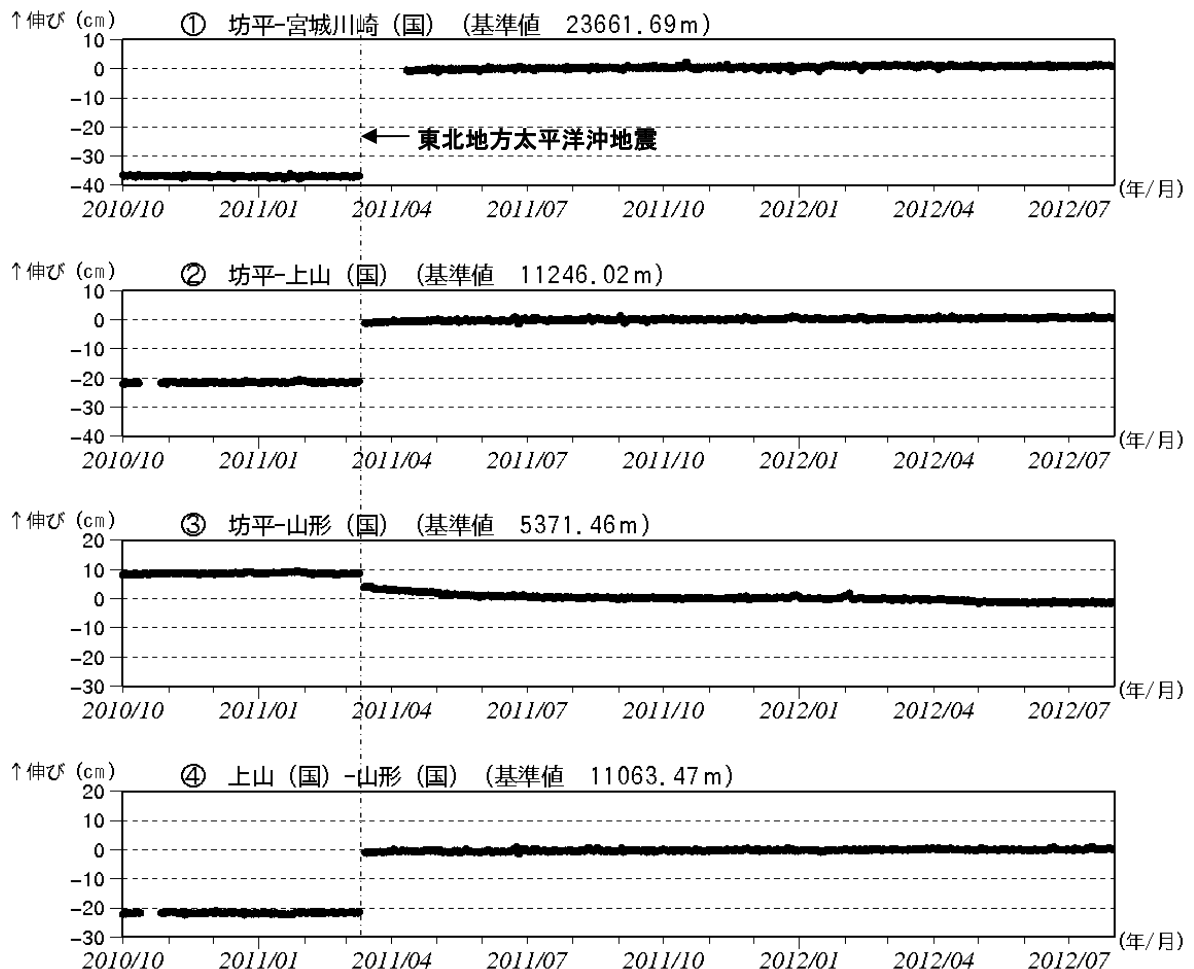
図5 蔵王山 GPS 基線長変化図 (2010 年 10 月～2012 年 7 月)
