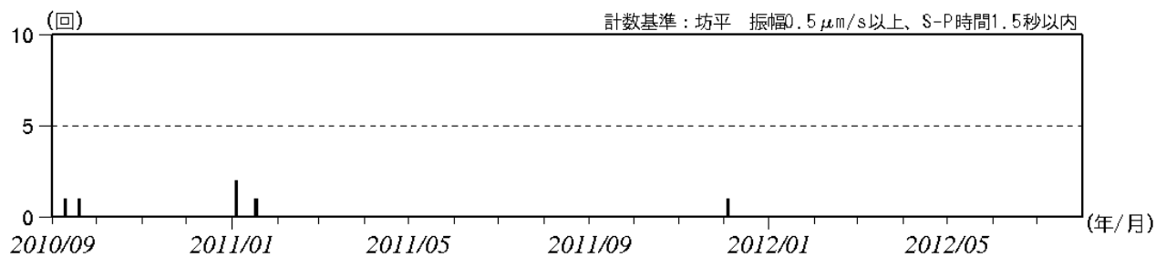
図3 蔵王山 火山性地震の日別回数（2010年9月～2012年7月）
