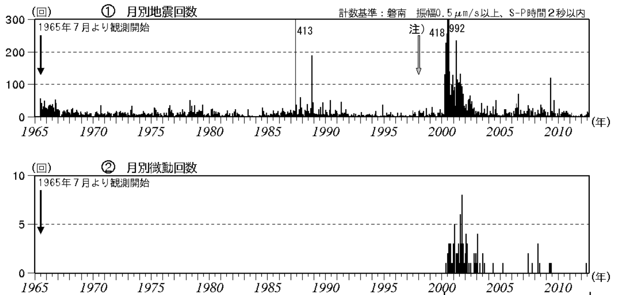
図 4※ 磐梯山 ①月別地震回数(1965 年 7 月～2012 年 8 月)
