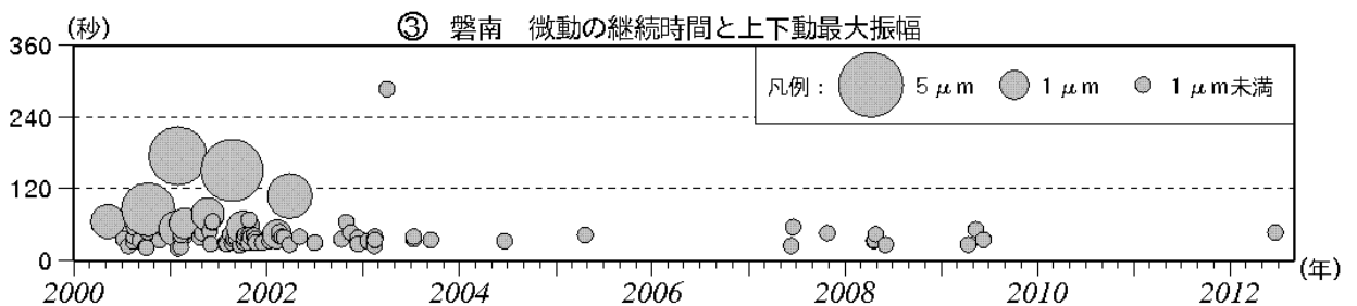
図 5※ 磐梯山 最近の地震と微動の活動経過図 (2000 年 1 月～2012 年 8 月)
