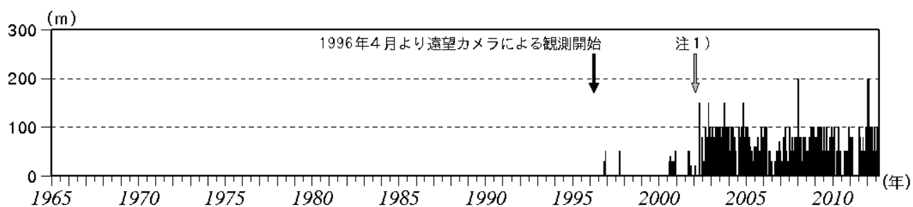
図 3 磐梯山 月最大噴気高（1996 年 4 月～2012 年 8 月）
