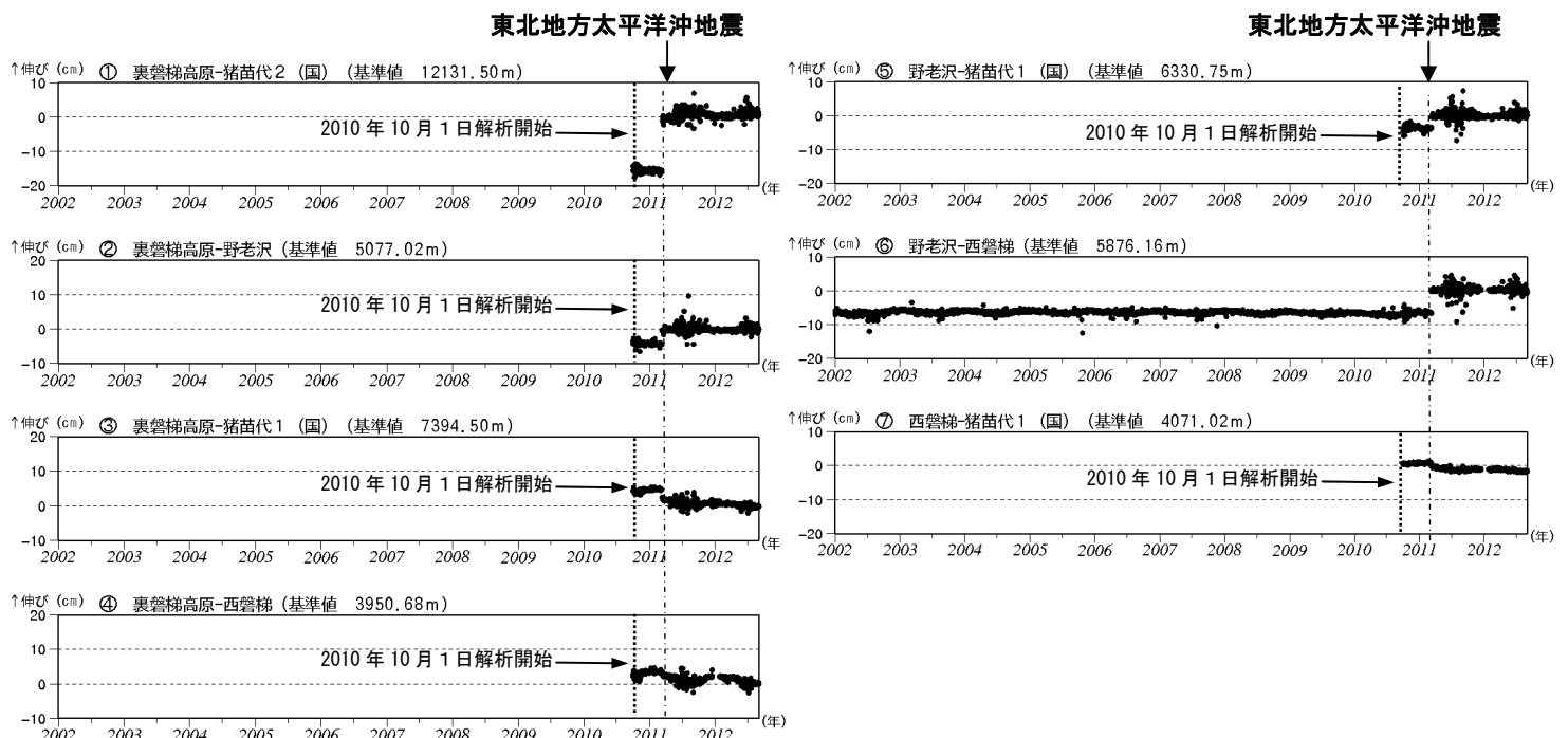
図7 磐梯山 GPS 基線長変化図（2002年1月～2012年8月）
