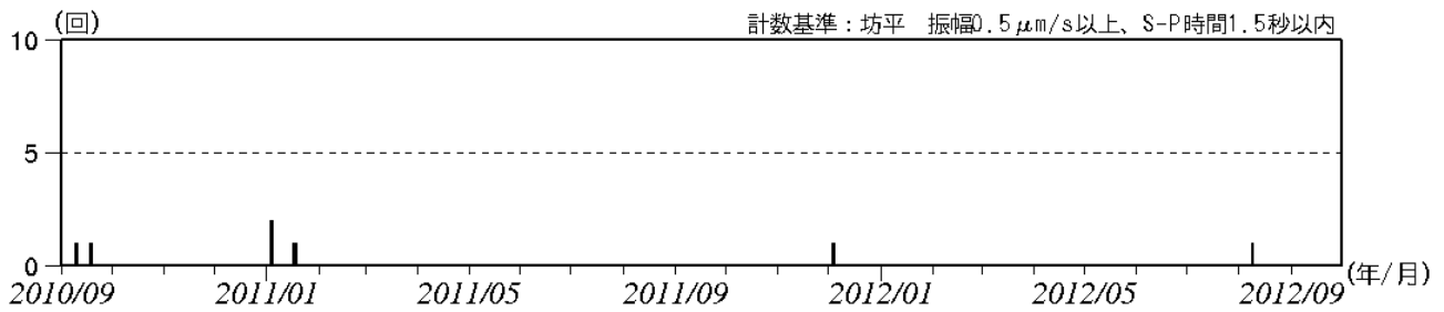
図 2 蔵王山 火山性地震の日別回数（2010 年 9 月～2012 年 9 月） 2010 年 9 月 1 日から観測開始。
