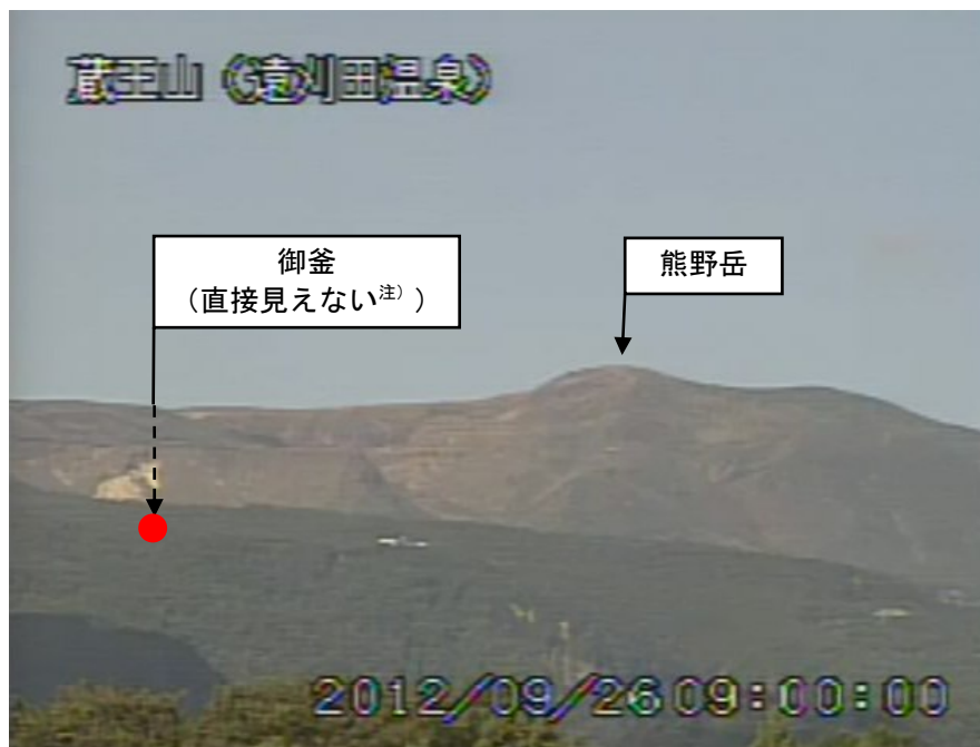
図 1 蔵王山 遠望カメラの映像（9 月 26 日 09 時 00 分頃）
