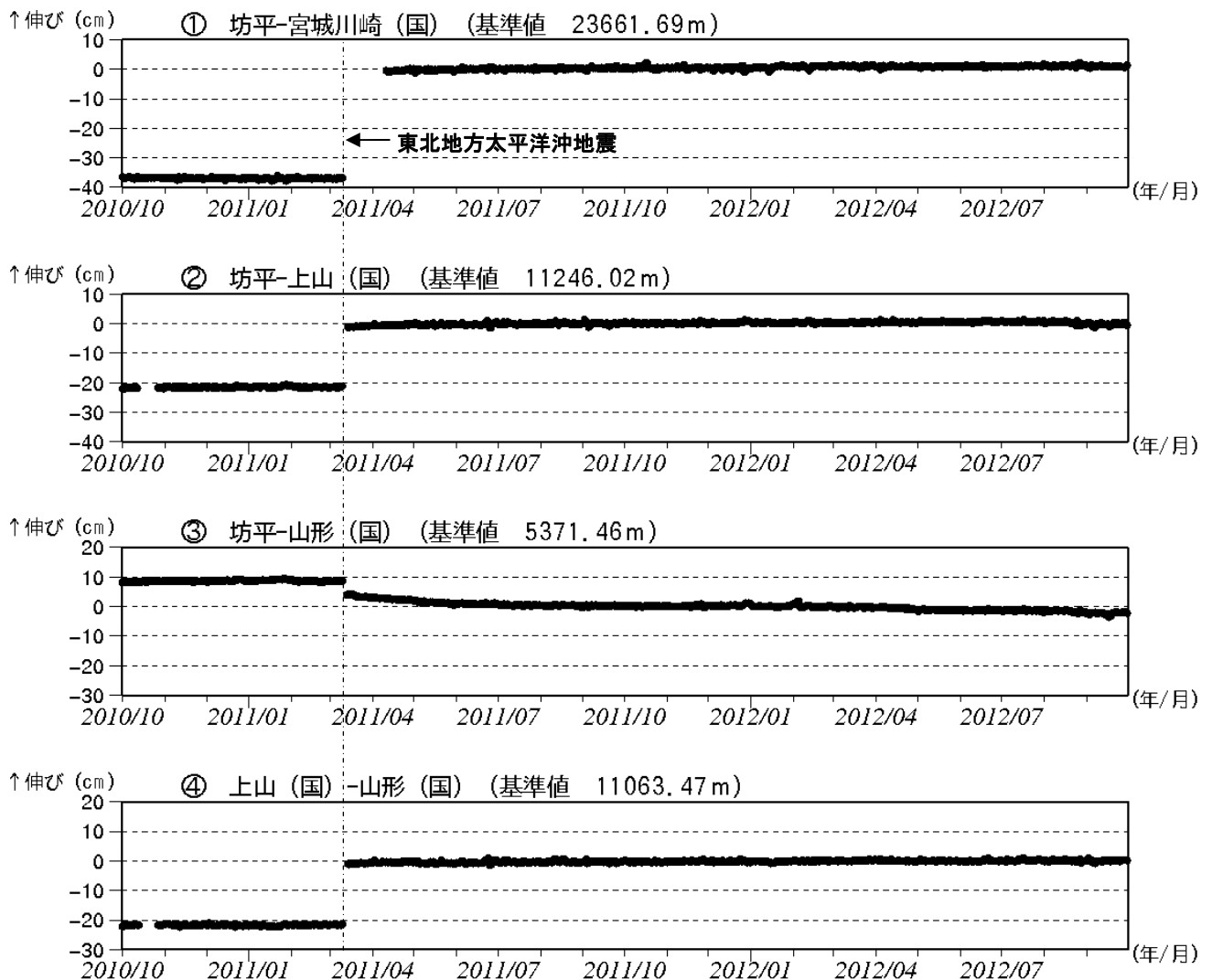
図 3※ 蔵王山 GPS 基線長変化図（2010 年 10 月～2012 年 9 月）
