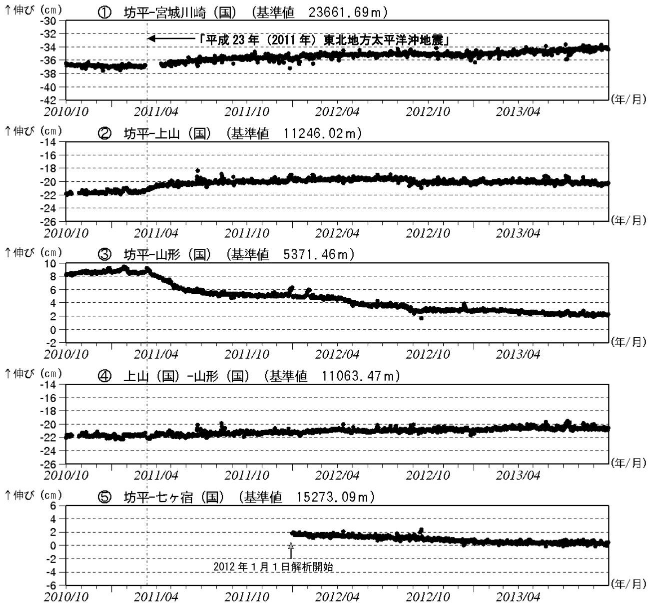
図 3 蔵王山 GPS 基線長変化図 (2010 年 10 月～2013 年 9 月)
