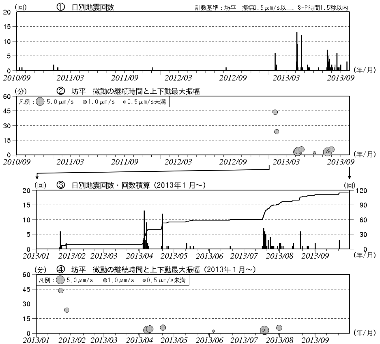
図2 蔵王山 火山活動経過図（2010年9月～2013年9月）
