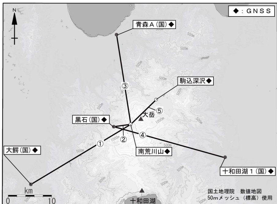
図 9 八甲田山 GNSS 観測点配置図
