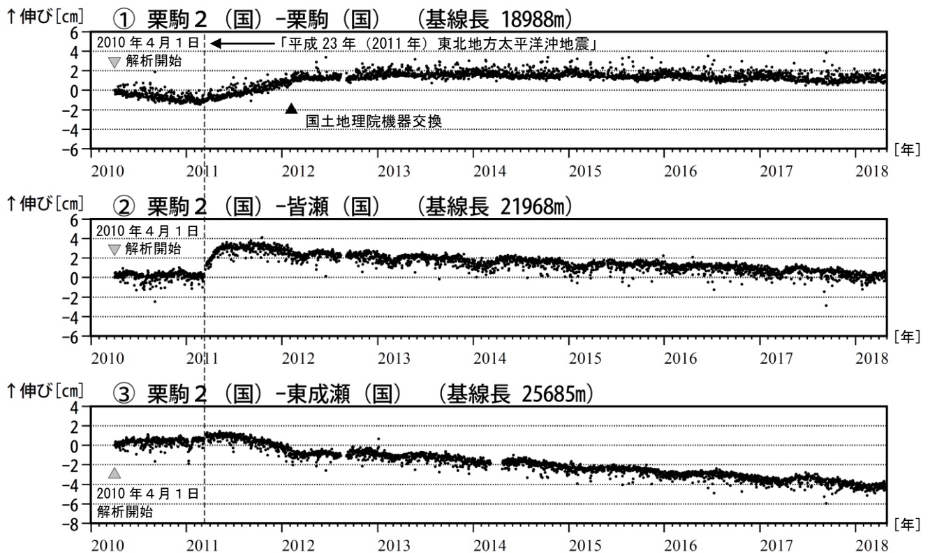
図4 栗駒山 GNSS 1) 基線長変化図（2010年4月～2018年4月）
