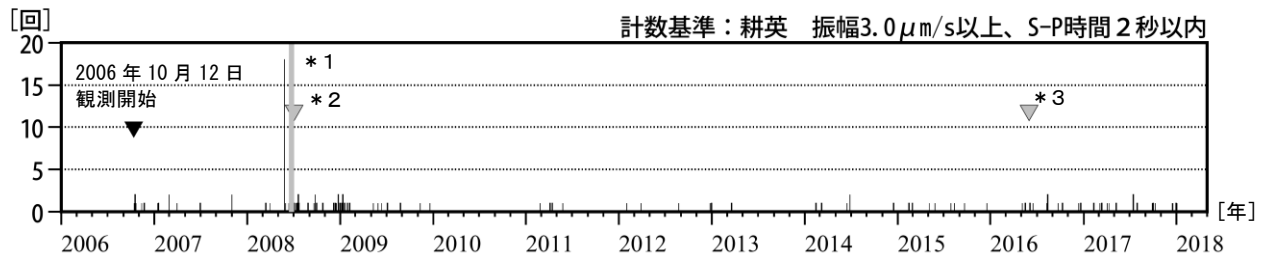
図3 栗駒山 日別地震回数（2006年10月～2018年4月）
