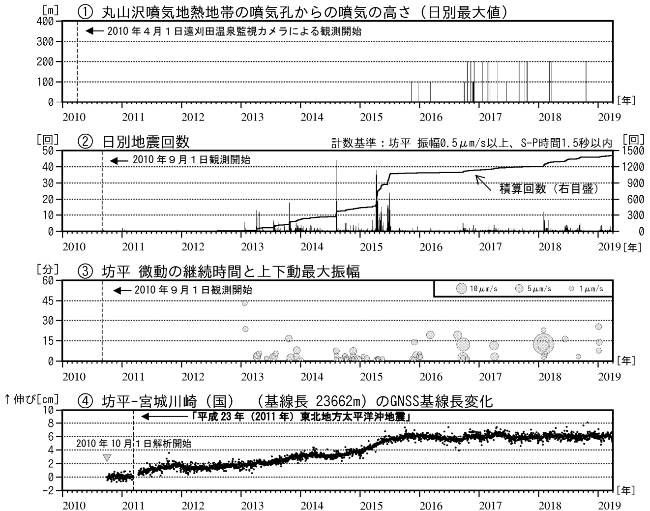
図 2 蔵王山 火山活動経過図（2010年 4 月～2019年 3 月）
