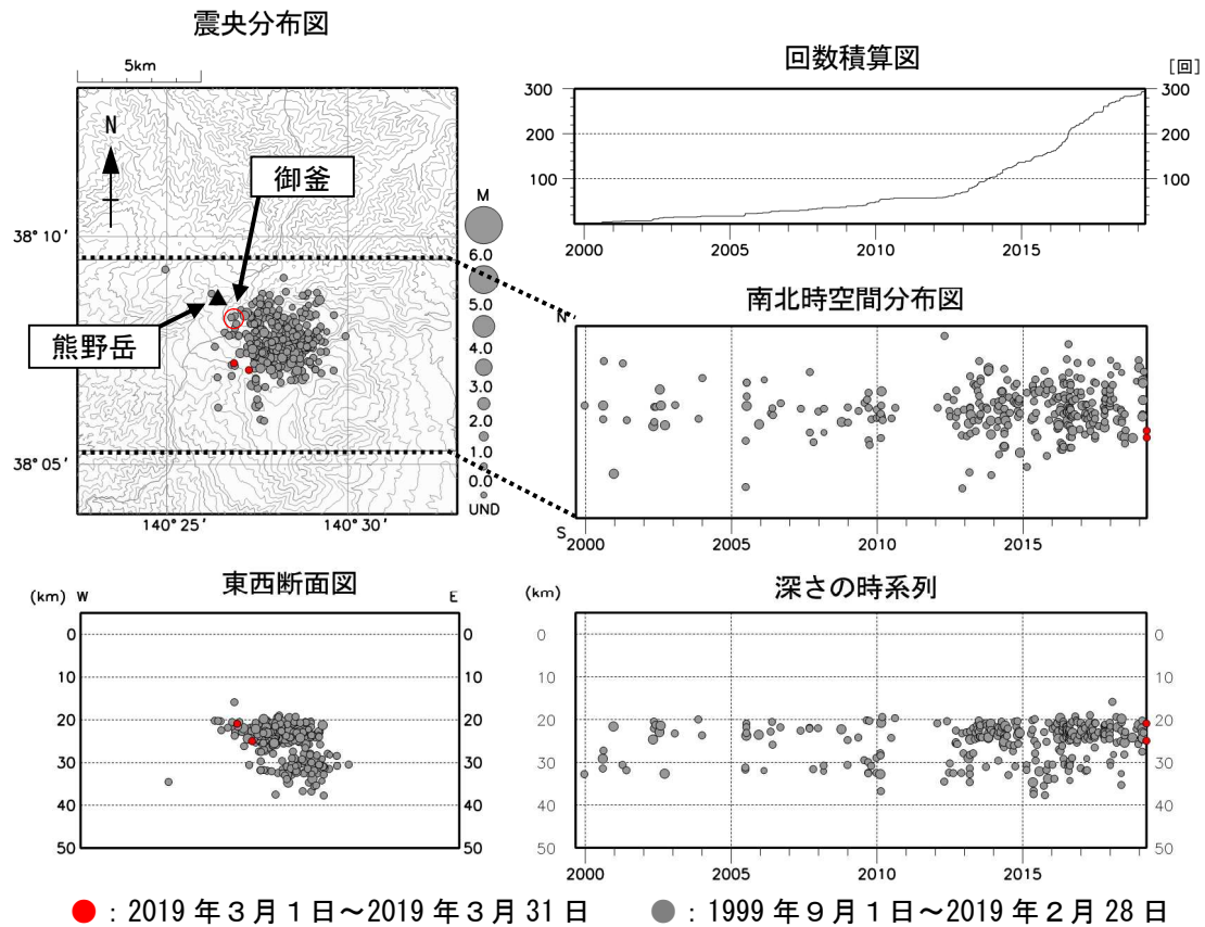
図 3 蔵王山 広域地震観測網による深部低周波地震活動（1999 年 9 月～2019 年 3 月）
