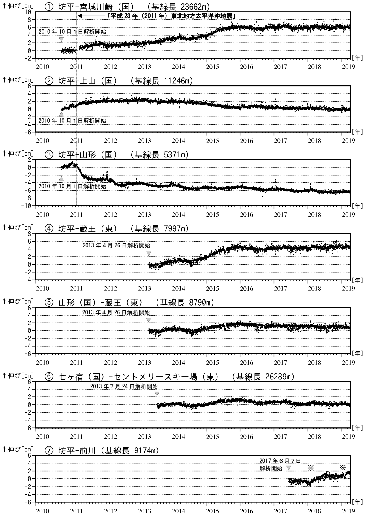
図 4 蔵王山 GNSS 基線長変化図 (2010 年 10 月～2019 年 3 月)
