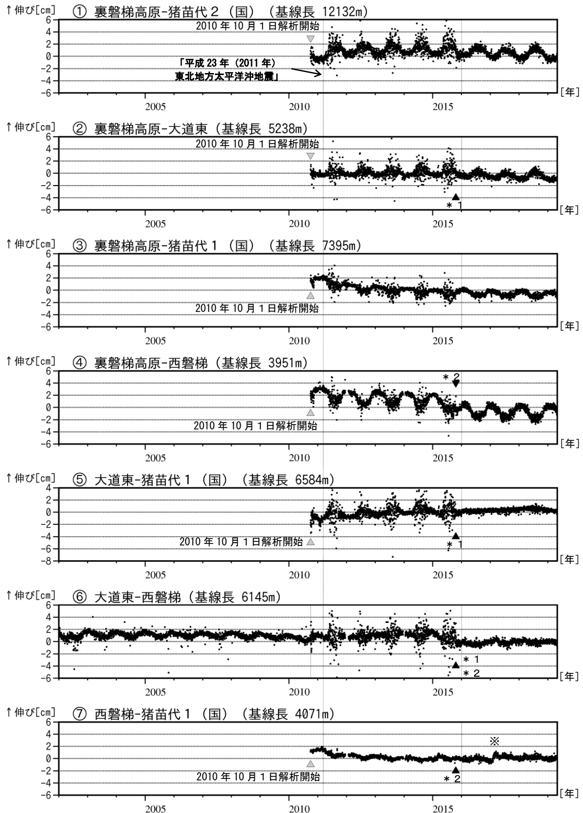
図 4 磐梯山 GNSS 基線長変化図 (2002 年 1 月～2019 年 4 月)
