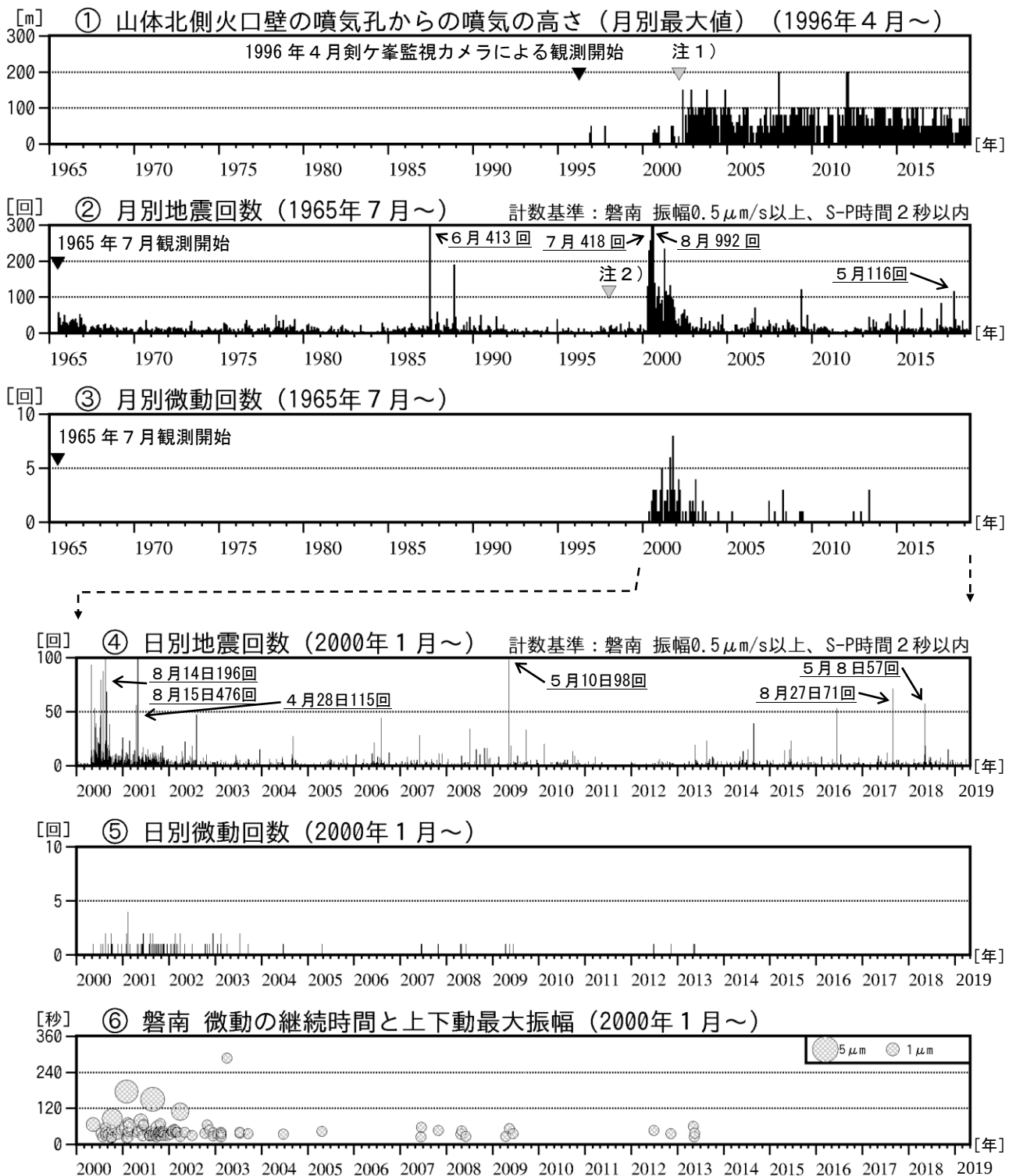
図3 磐梯山 火山活動経過図（1965年7月～2019年4月）
