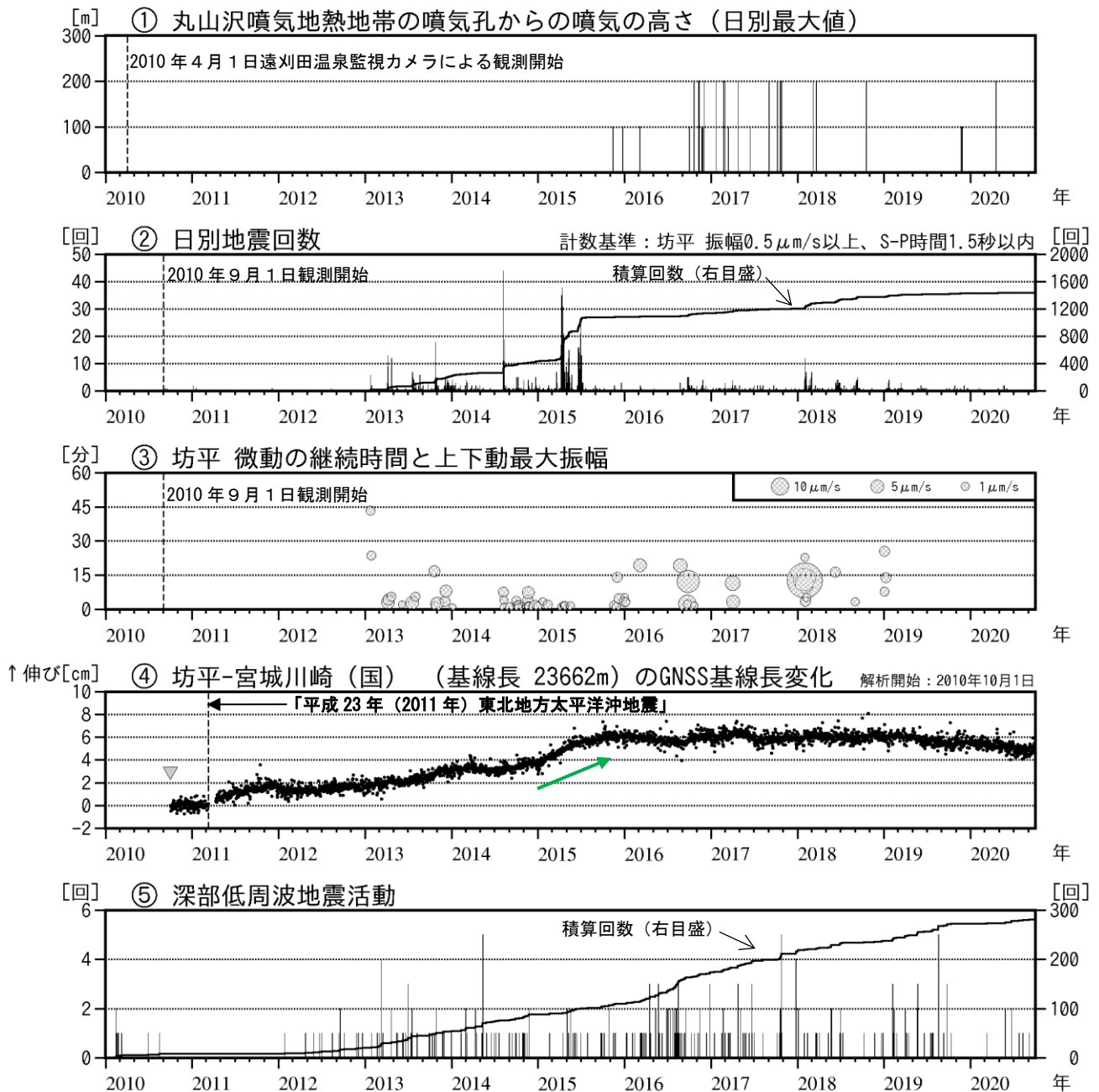
図3 蔵王山 火山活動経過図（2010年4月～2020年9月）
