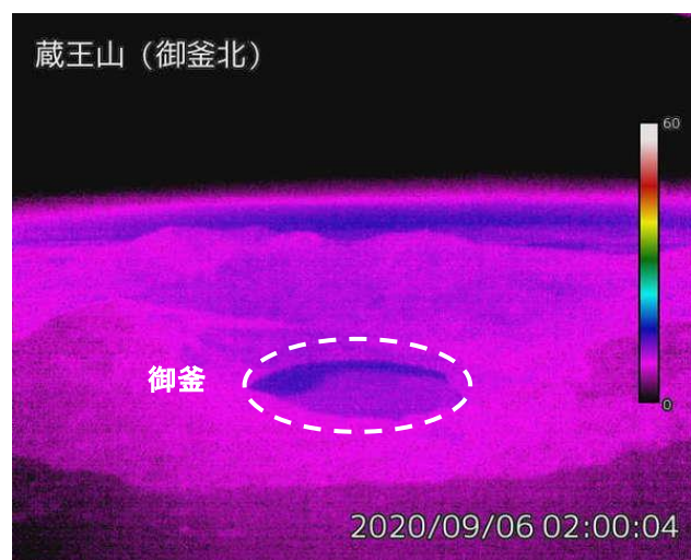
図2 蔵王山 山頂部の地表面温度分布（9月6日）
