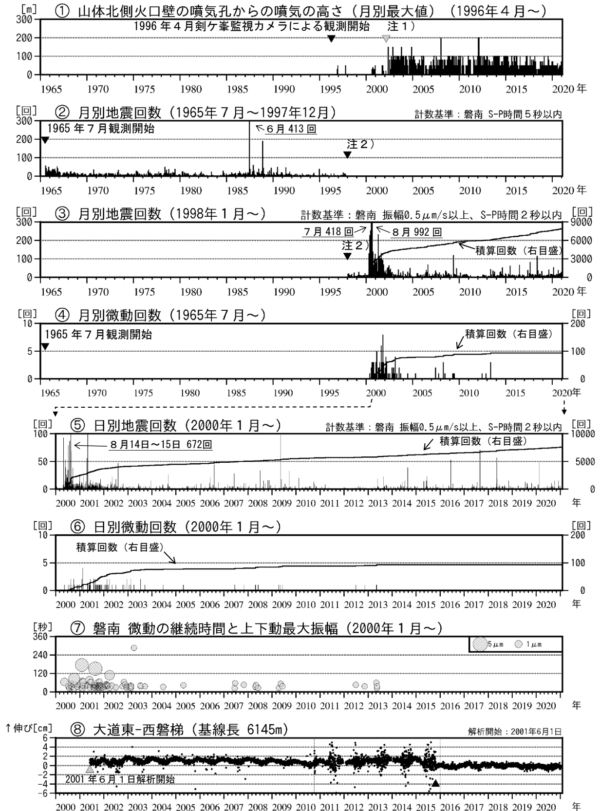
図3 磐梯山 火山活動経過図（1965年7月～2021年1月）
