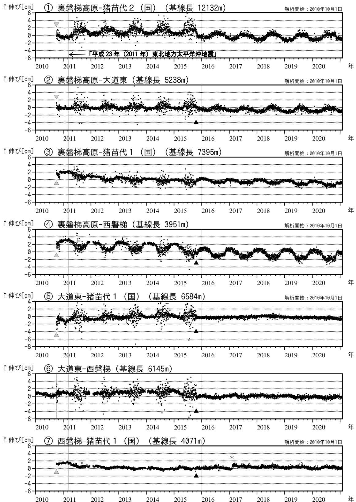
図4 磐梯山 GNSS 基線長変化図 (2010年1月～2021年1月)
