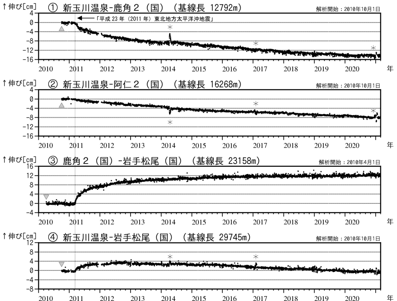
図4 秋田焼山 GNSS 基線長変化図（2010年4月～2021年2月）
