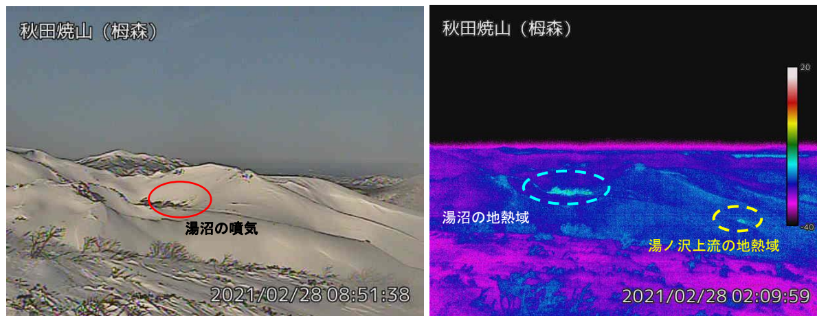
図2 秋田焼山 湯沼と湯ノ沢上流の状況（2月28日）と地表面温度分布（2月28日）
