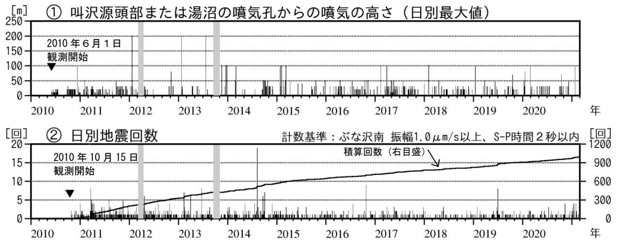
図3 秋田焼山 火山活動経過図（2010年6月～2021年2月）
