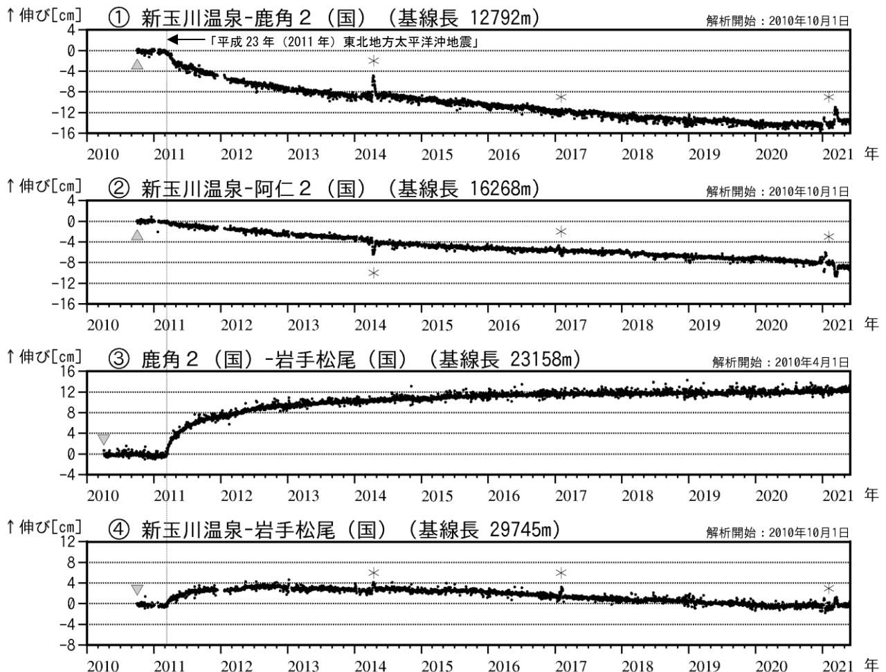
図4 秋田焼山 GNSS 基線長変化図（2010年4月～2021年5月）
