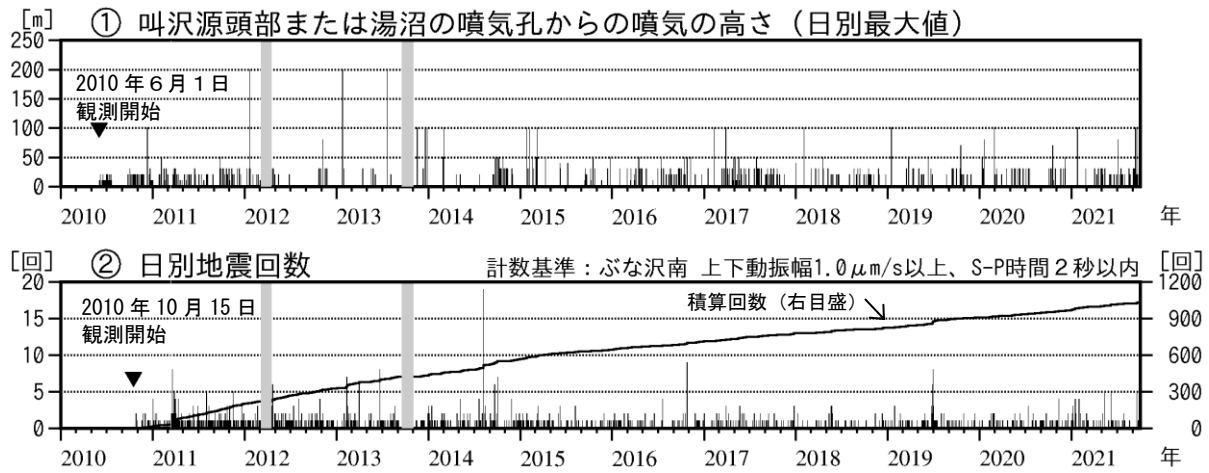
図3 秋田焼山 火山活動経過図（2010年6月～2021年9月）
