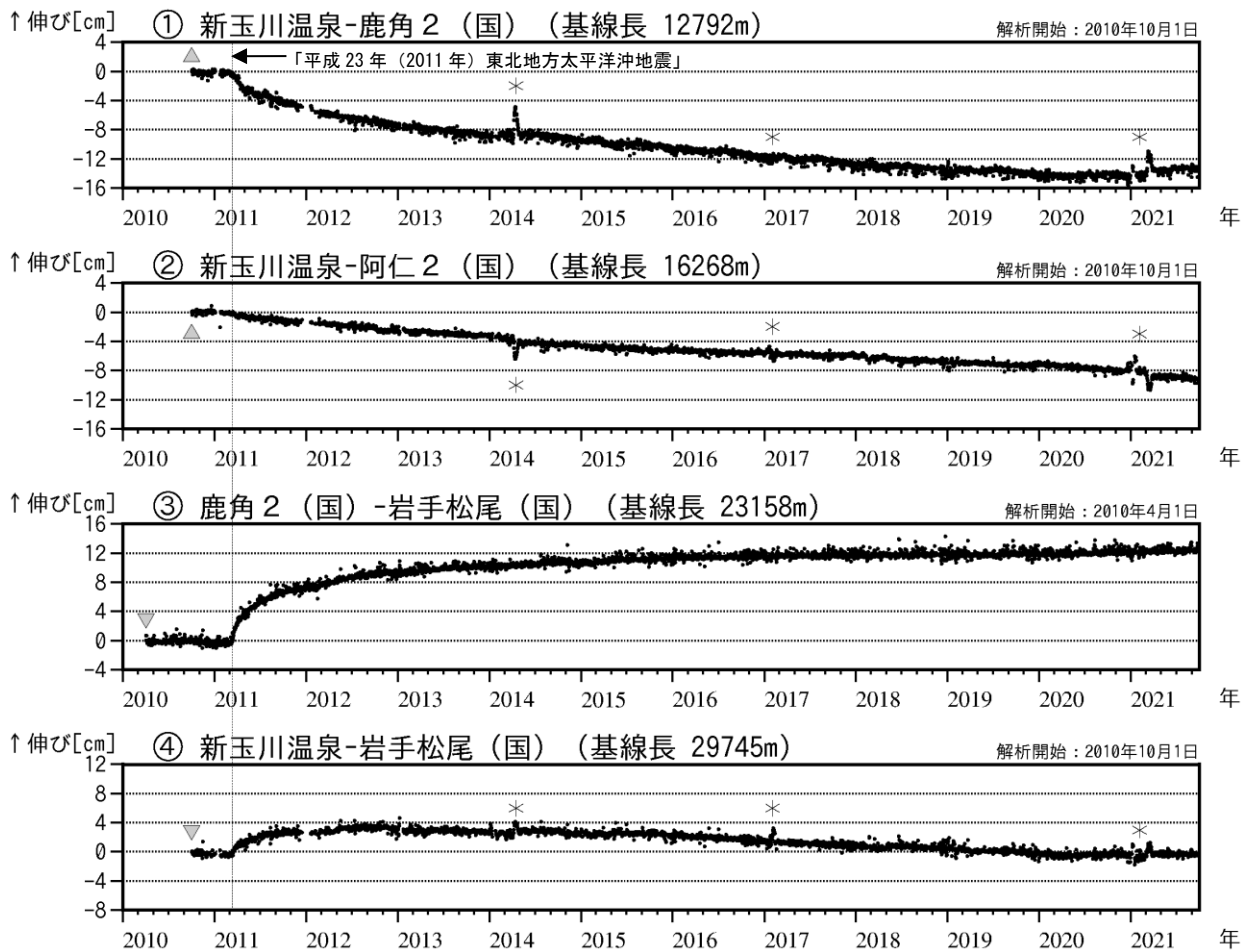
図4 秋田焼山 GNSS 基線長変化図（2010年4月～2021年9月）
