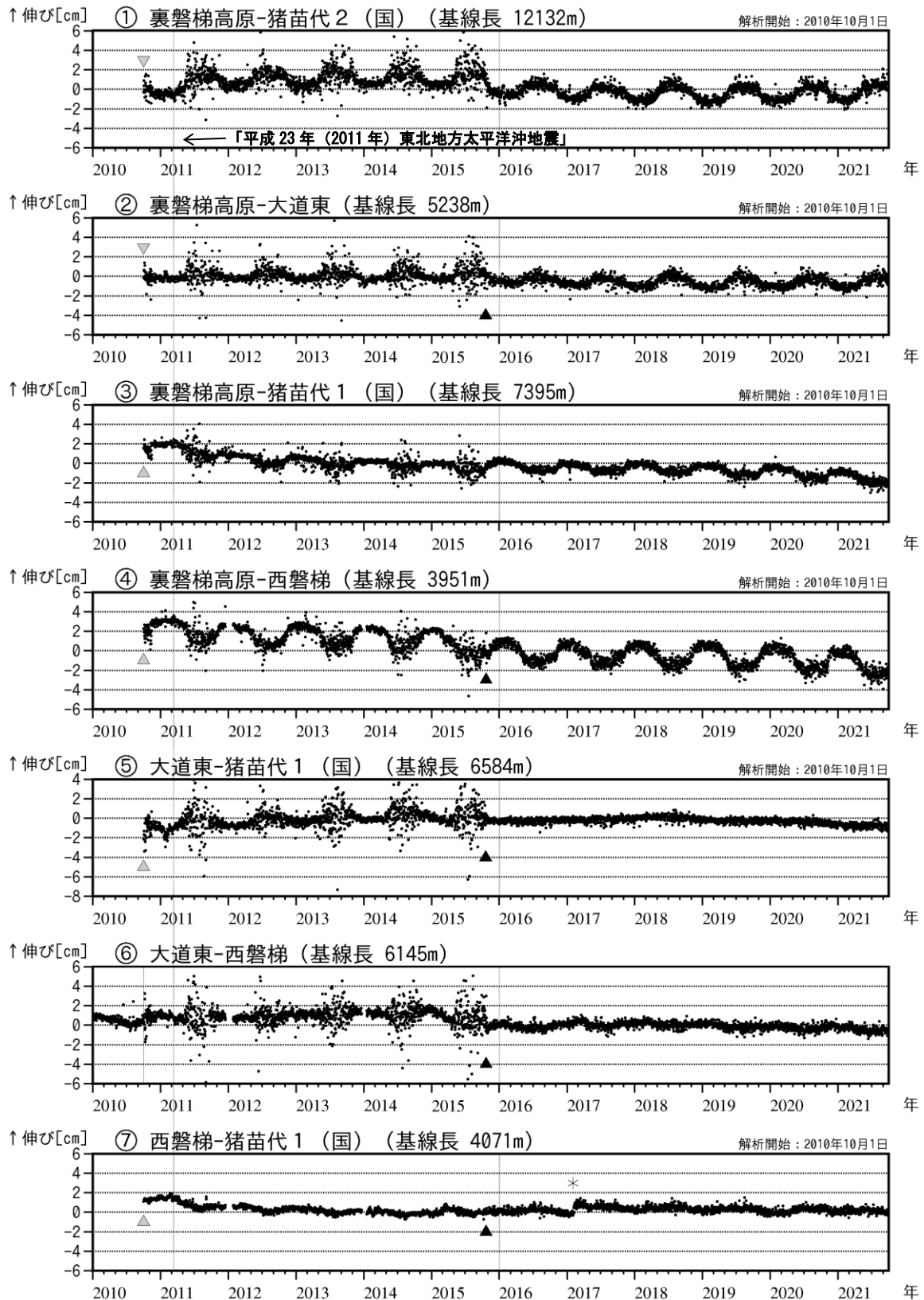
図4 磐梯山 GNSS 基線長変化図 (2010年1月～2021年9月)
