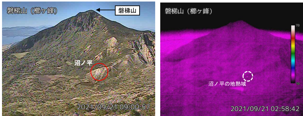
図2 磐梯山 沼ノ平周辺の状況と地表面温度分布（9月21日）
