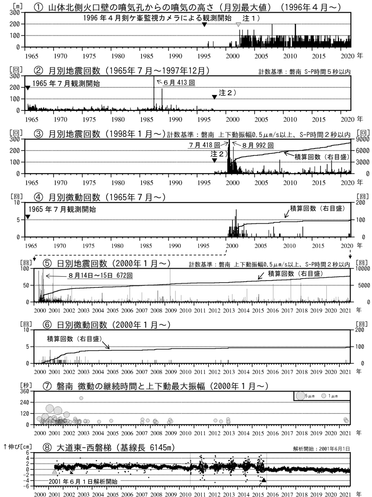
図3 磐梯山 火山活動経過図（1965年7月～2021年9月）
