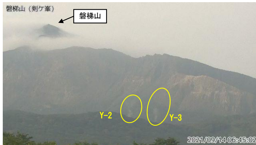
図1 磐梯山 山体北側火口壁の噴気の状況（9月14日）
