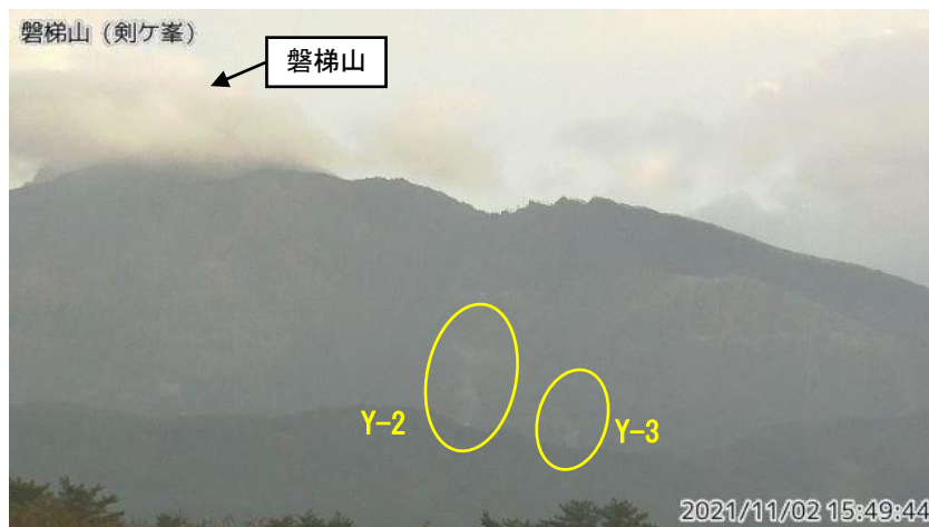
図1 磐梯山 山体北側火口壁の噴気の状況（11月2日）
