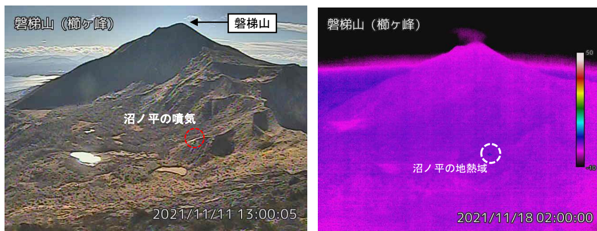
図2 磐梯山 沼ノ平周辺の状況（11月11日）と地表面温度分布（11月18日）
