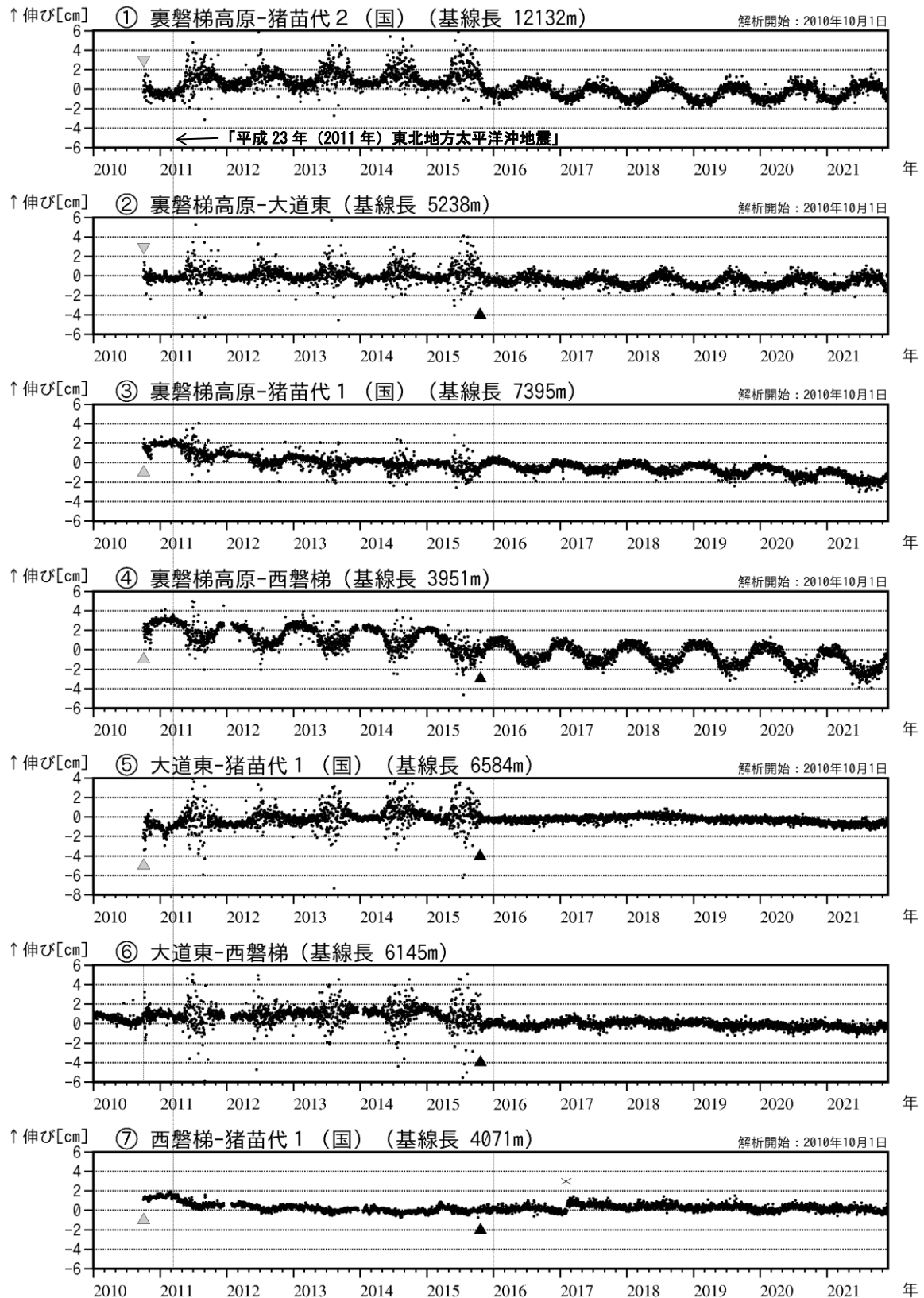
図4 磐梯山 GNSS 基線長変化図 (2010年1月～2021年11月)
