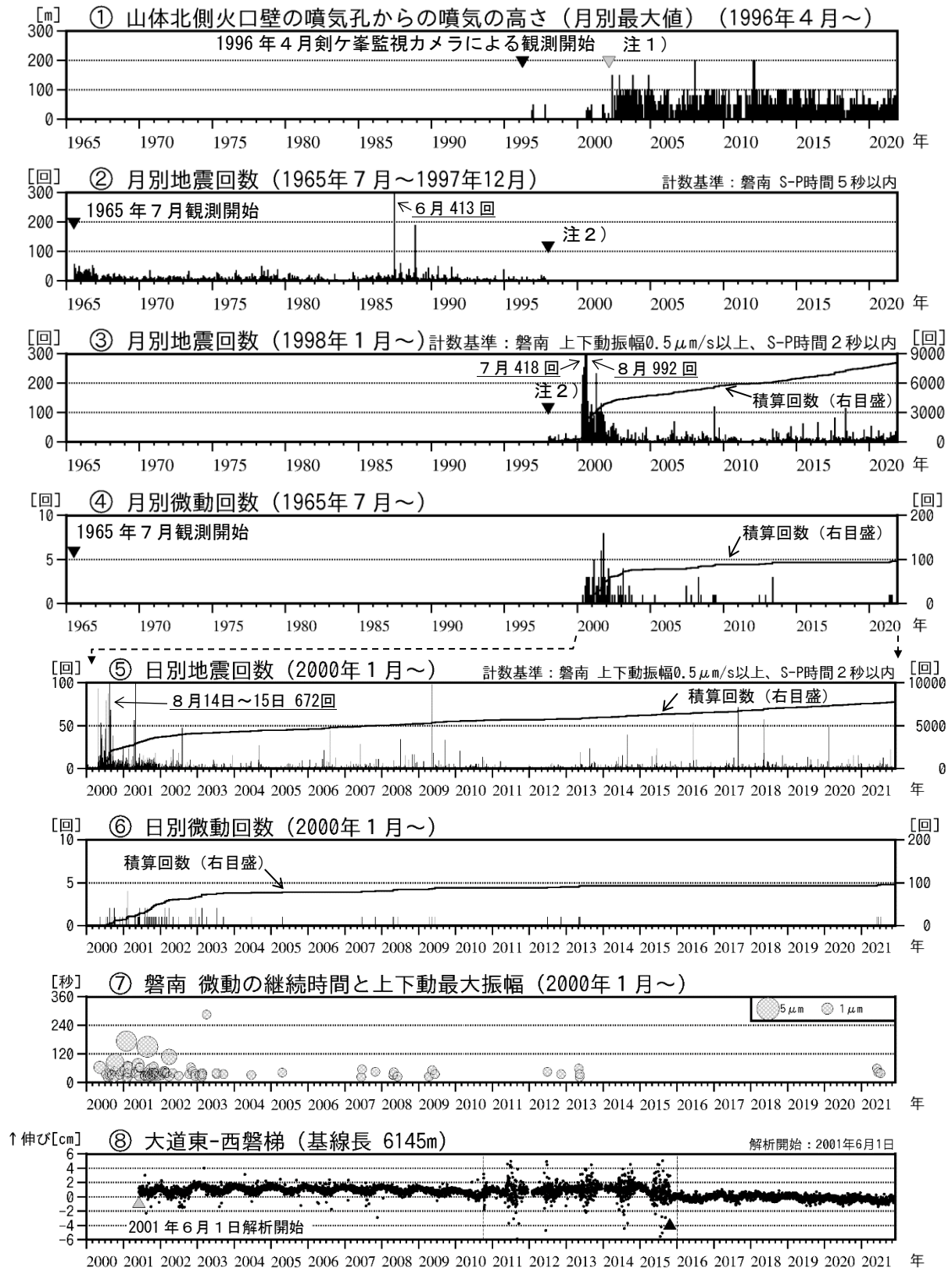
図3 磐梯山 火山活動経過図（1965年7月～2021年11月）
