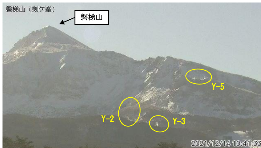
図1 磐梯山 山体北側火口壁の噴気の状況（12月14日）
