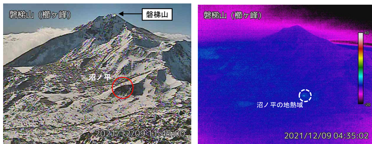
図2 磐梯山 沼ノ平周辺の状況と地表面温度分布（12月9日）
