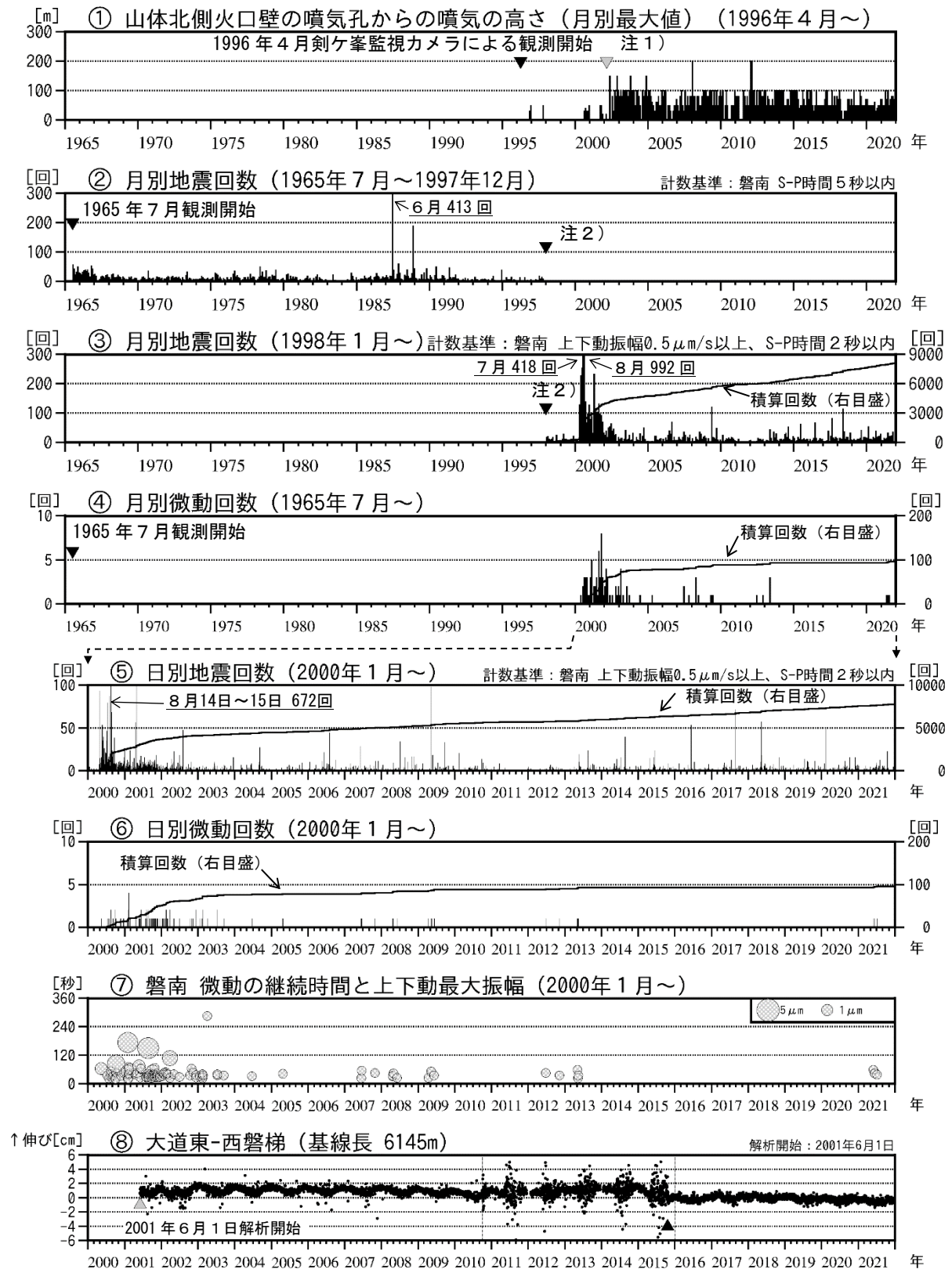
図3 磐梯山 火山活動経過図（1965年7月～2021年12月）
