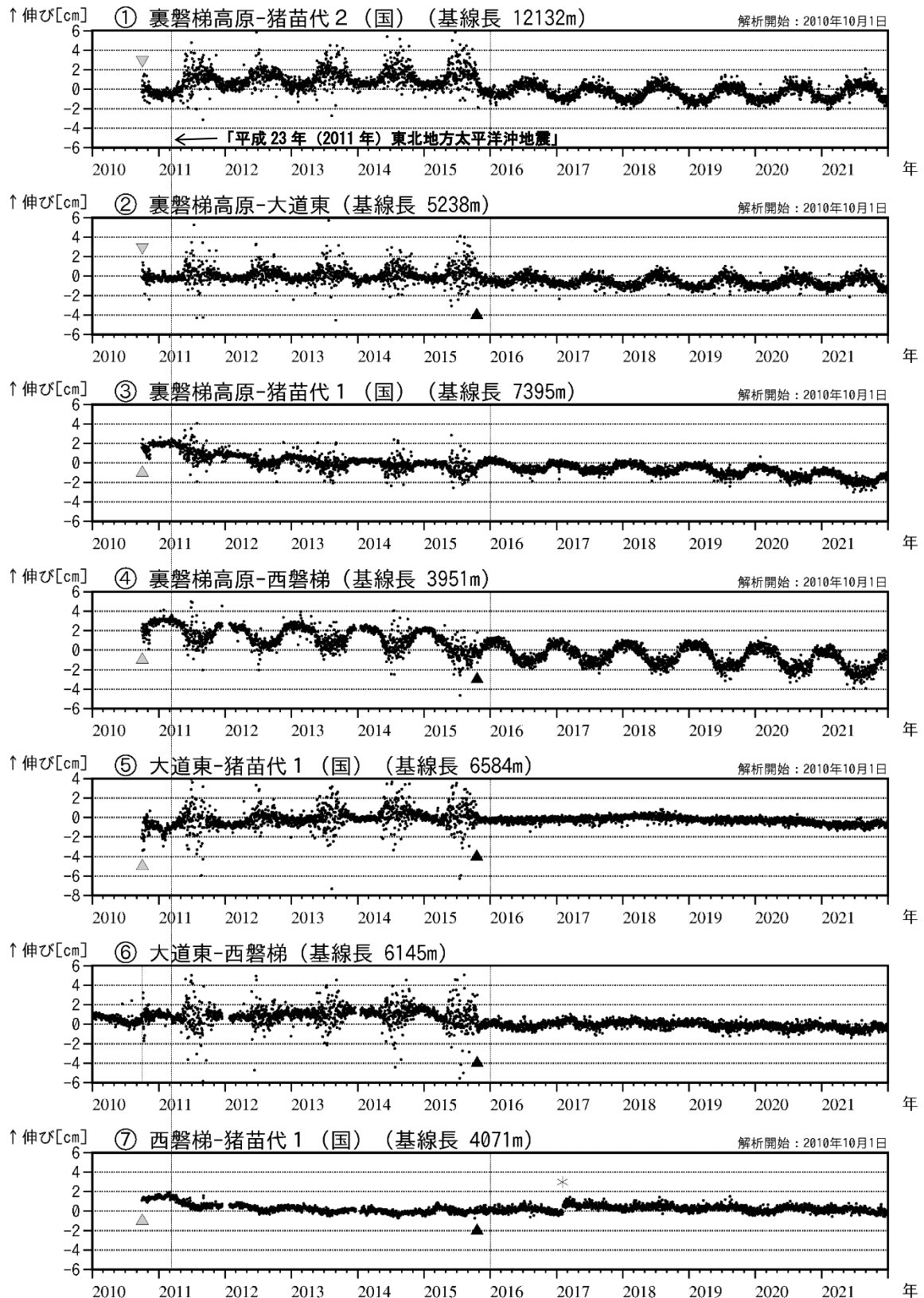
図4 磐梯山 GNSS 基線長変化図 (2010年1月～2021年12月)
