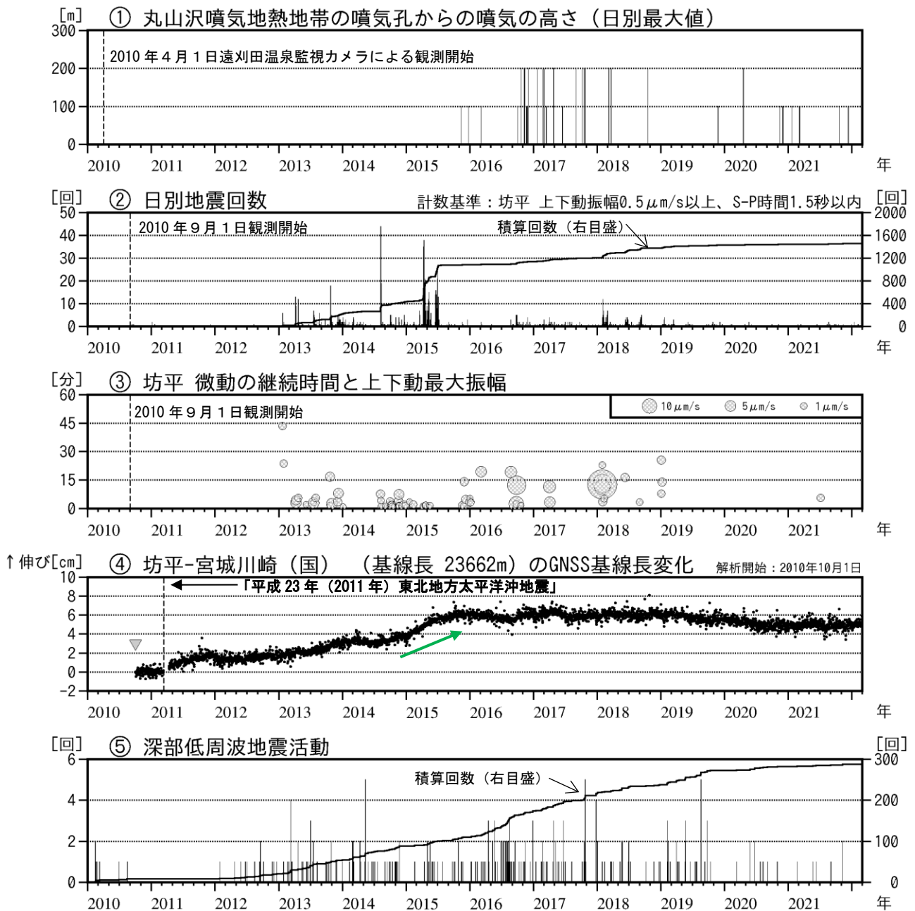
図2 蔵王山 火山活動経過図（2010年4月～2022年2月）
